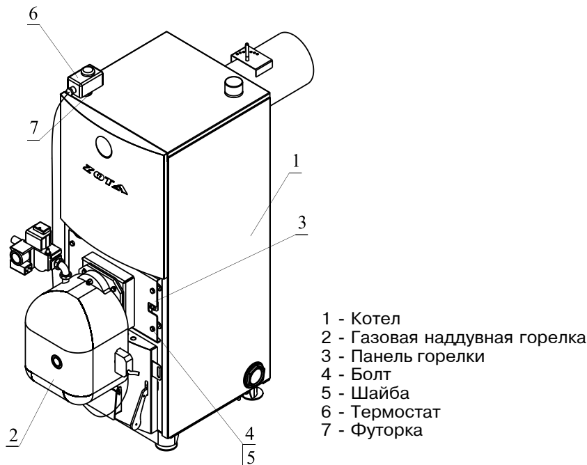
Рис.3 Котлы КСТ – 20...50Гн
