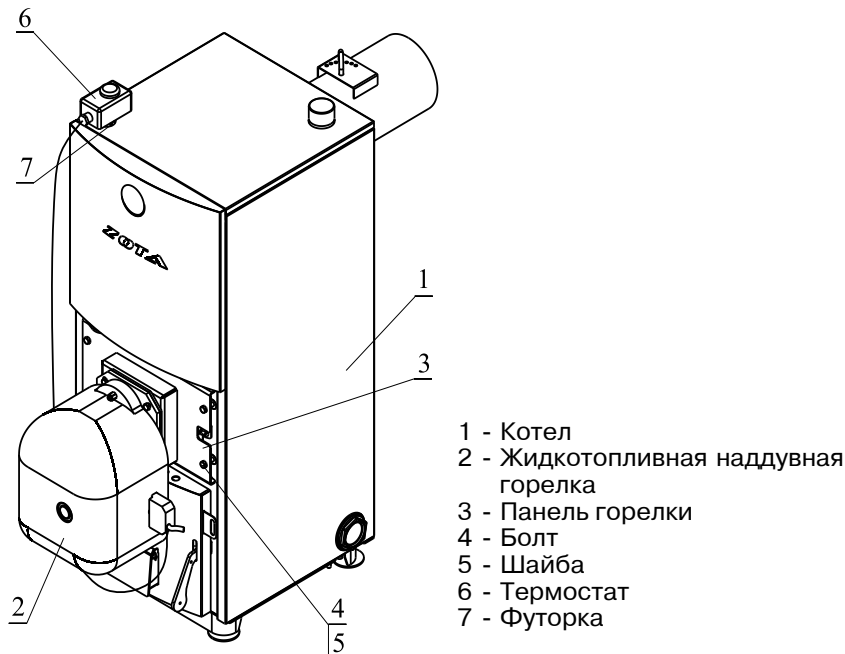
Рис.4 Котлы КСТ – 20...50Дт
