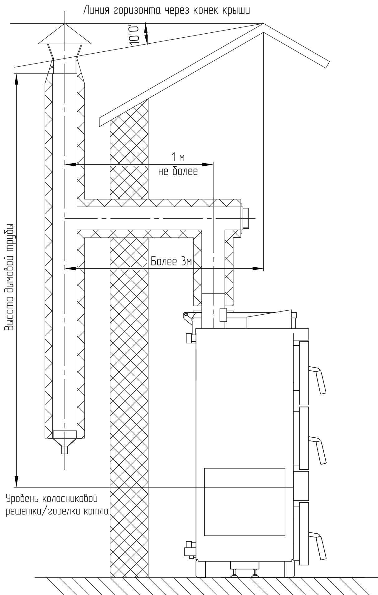
Рис.7.1 Варианты установки дымовой трубы с вертикальным дымовым патрубком
