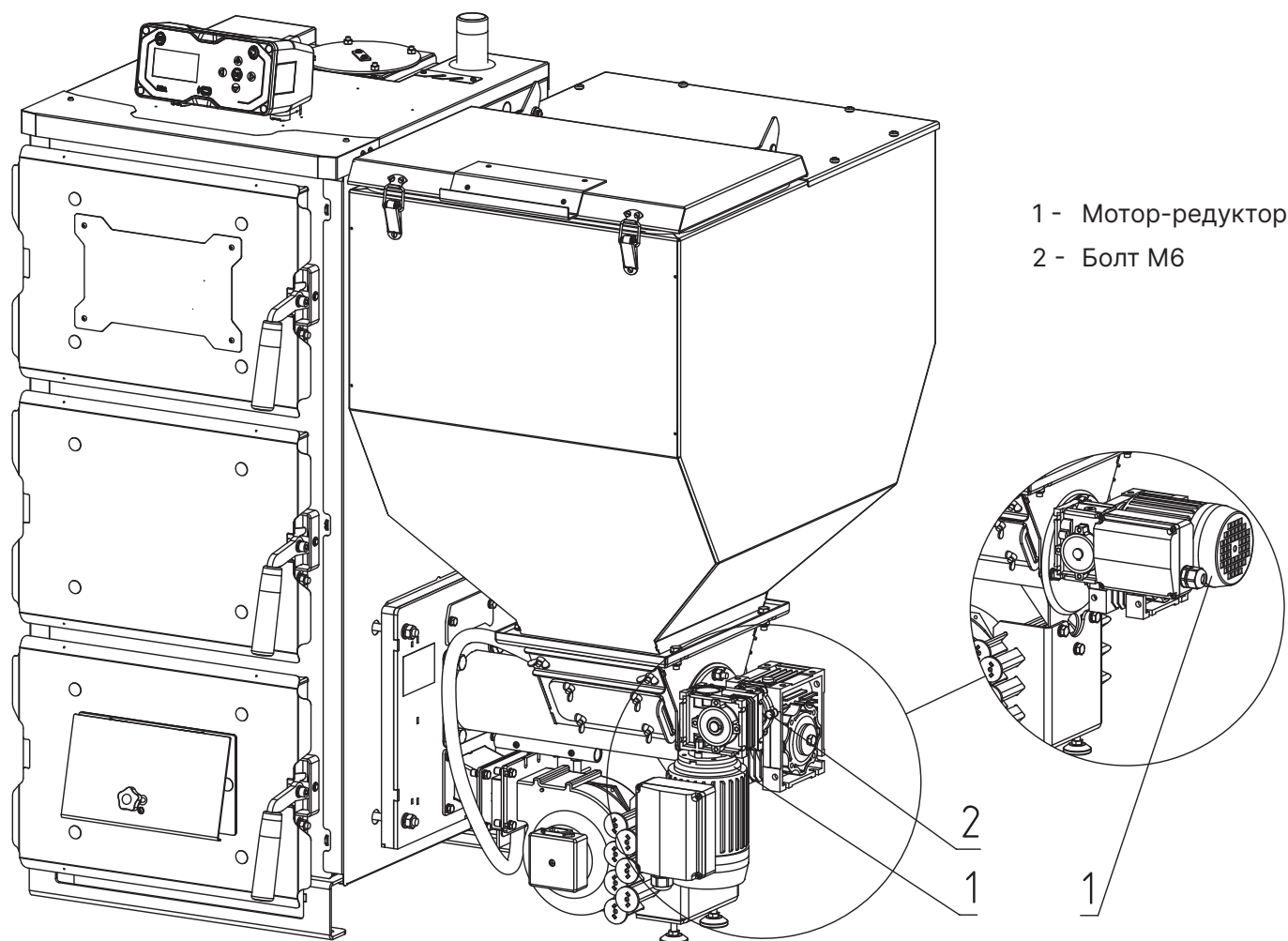
Рис.8 Изменение положение мотор-редуктора
