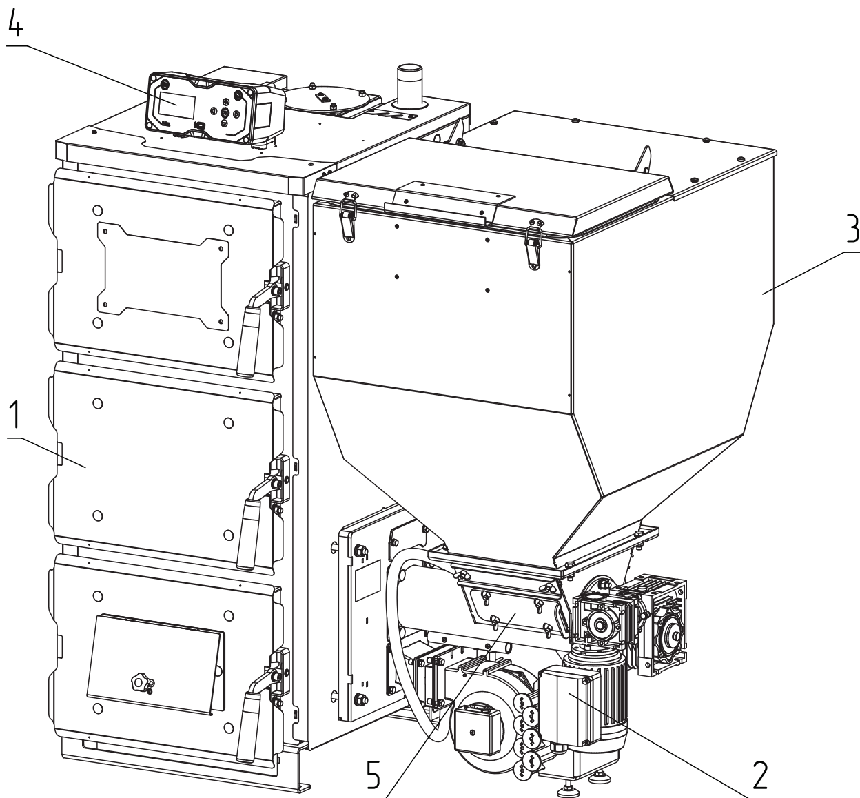
Рис.1 Конструкция котла ZOTA «Forta-R»
