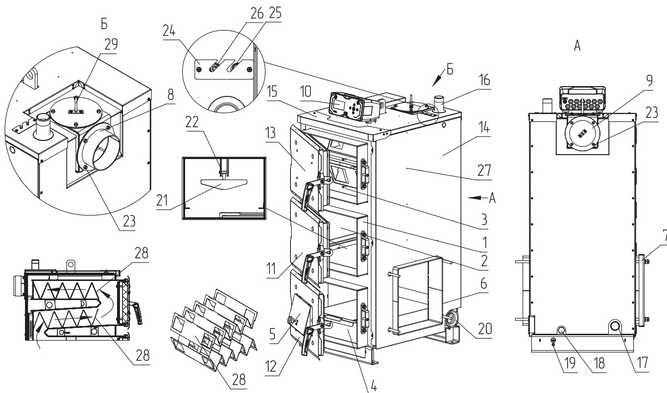
Рис.2 Конструкция теплообменника котла ZOTA «Forta-R»
