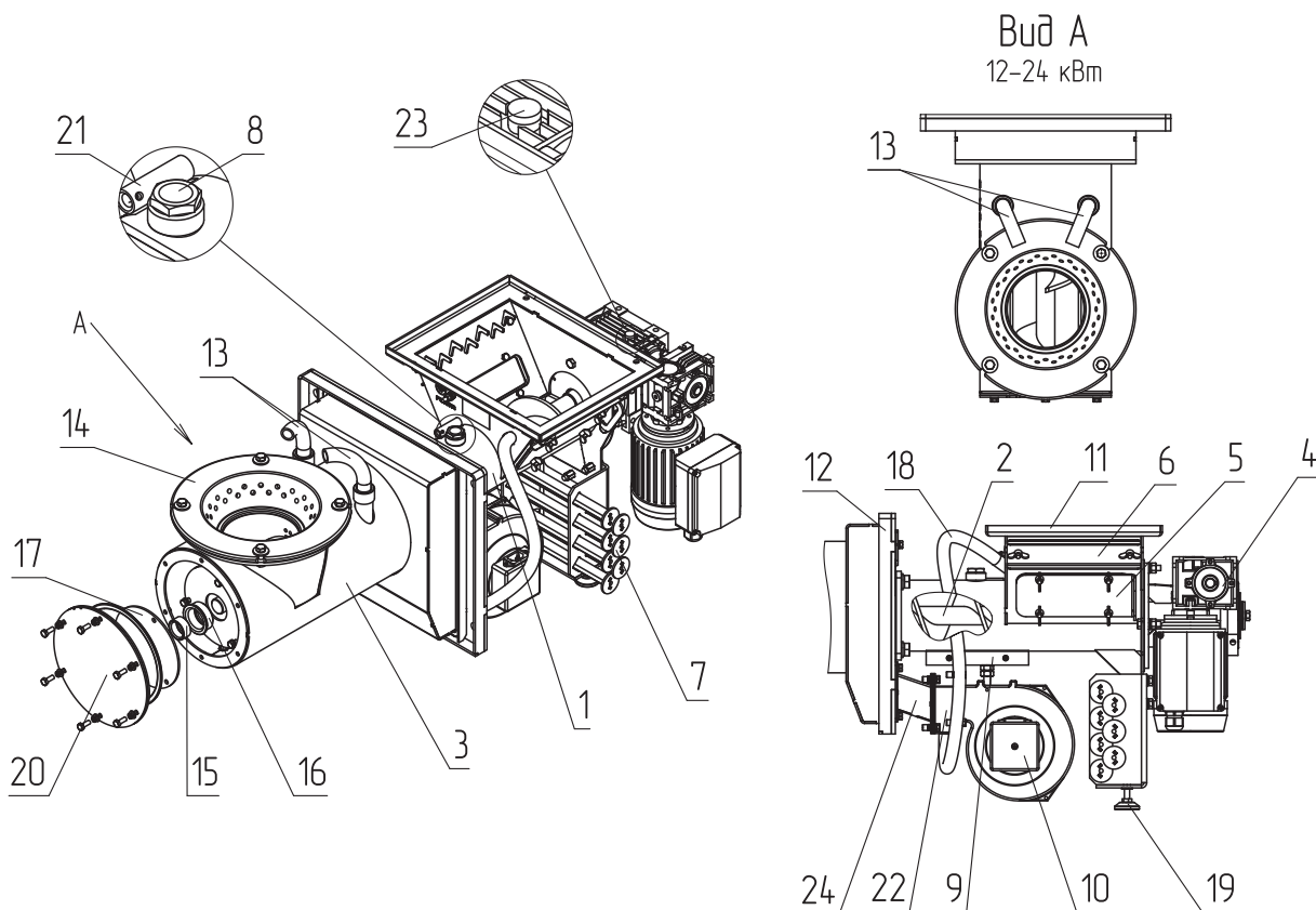
Рис.3 Механизм подачи топлива с горелкой котла
