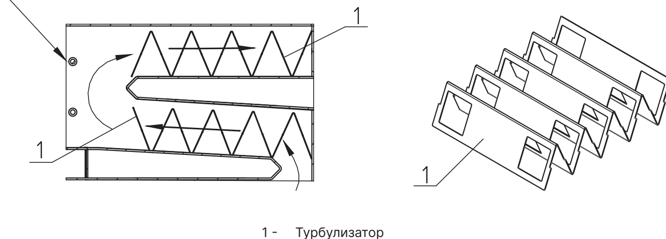
Рис.10 Установка турбулизаторов
