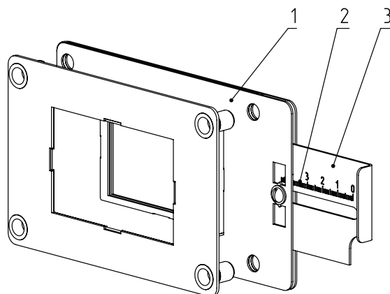
Рис.12 Заслонка вентилятора
