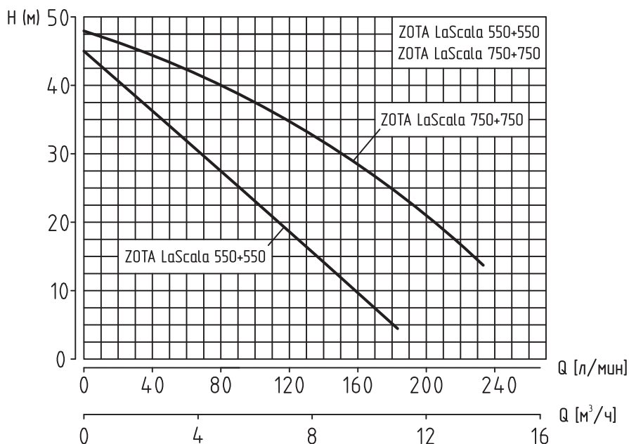
Рис. 11 Диаграммы напорно-расходных характеристик насосных станций
