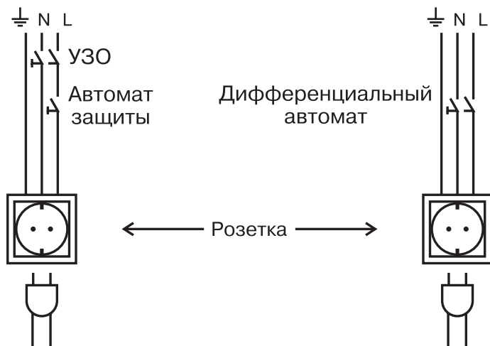
Рис. 8 Схема подключения насосной станции к электрической сети
