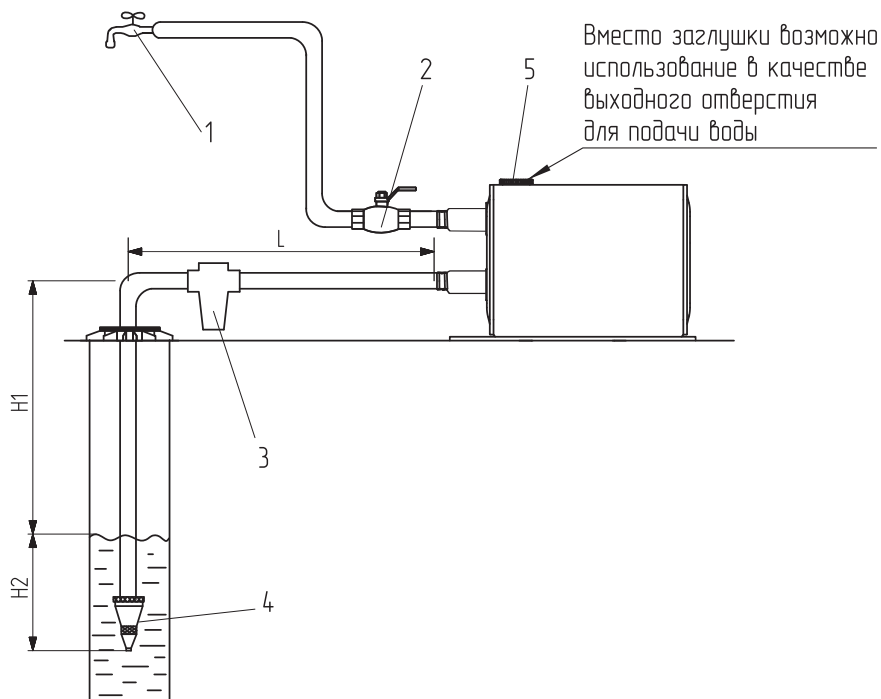
Рис. 6 Пример схемы монтажа насосной станции с подачей жидкости из колодца/ скважины
