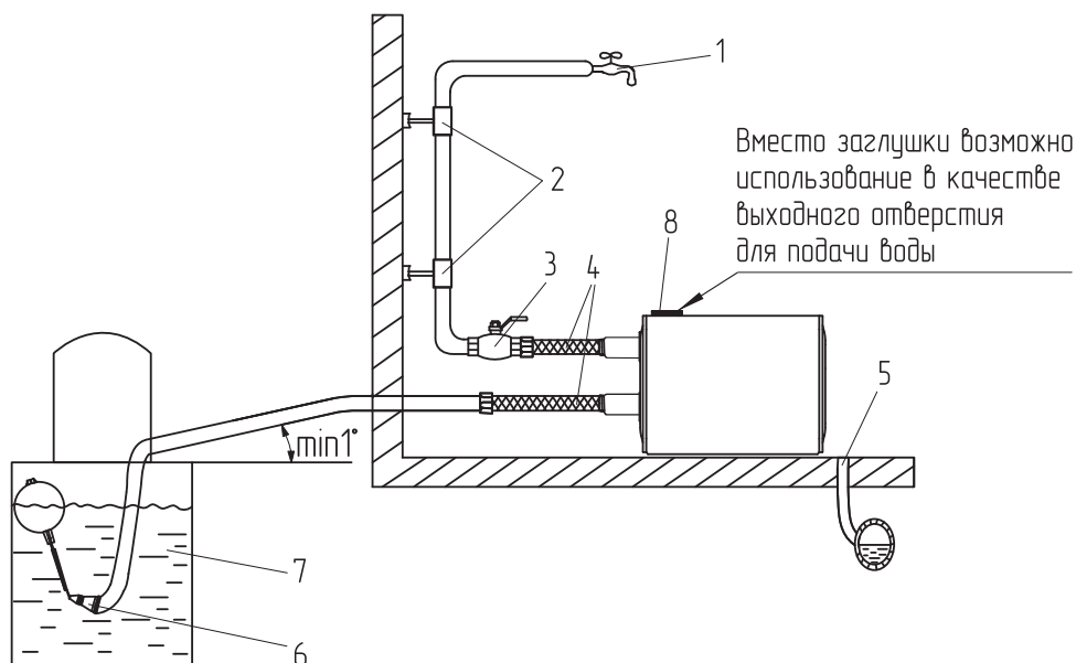
Рис. 7 Пример схемы монтажа насосной станции с подачей жидкости из резервуара
