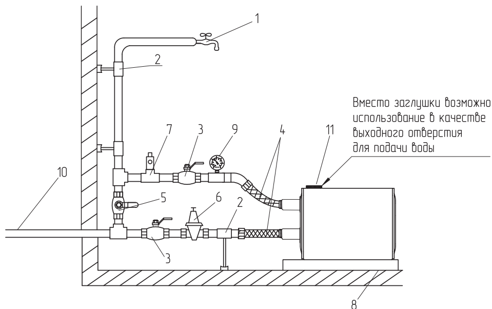
Рис. 5 Пример схемы монтажа для повышения давления воды из магистрального трубопровода
