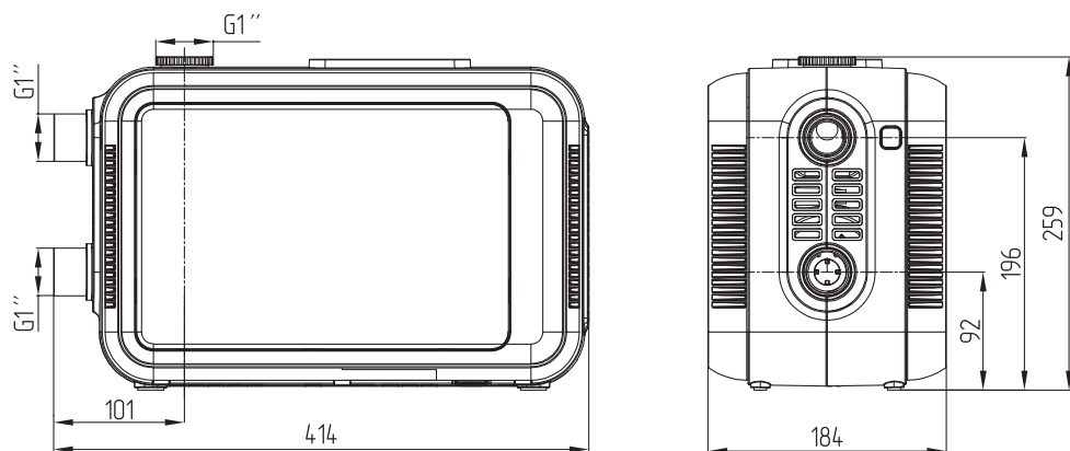
Рис. 4 Габаритные размеры насосной станции ZOTA LaScala
