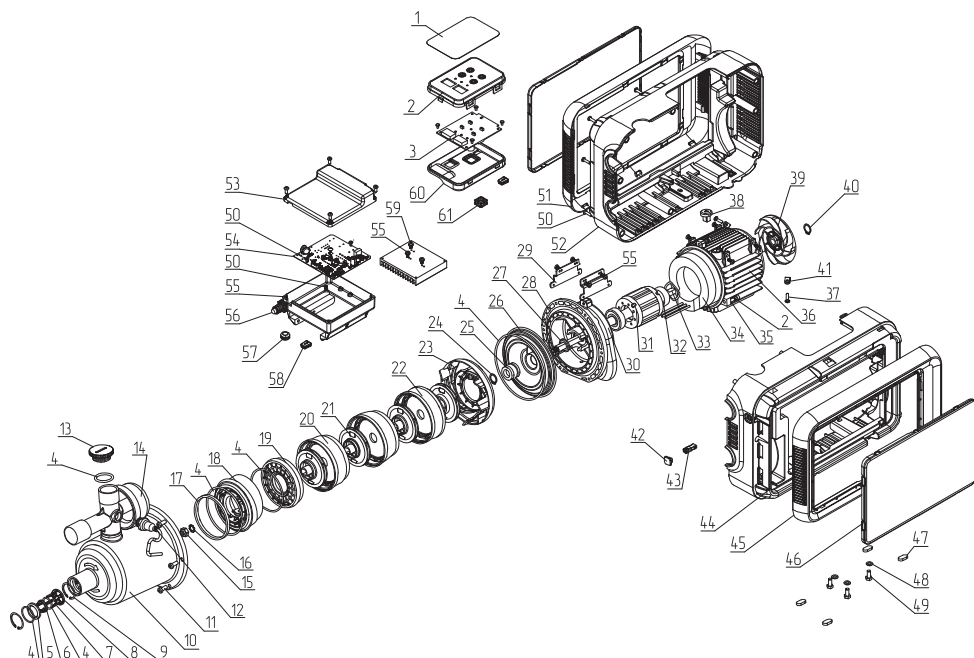
Рис. 3 Устройство насосной станции ZOTA LaScala
