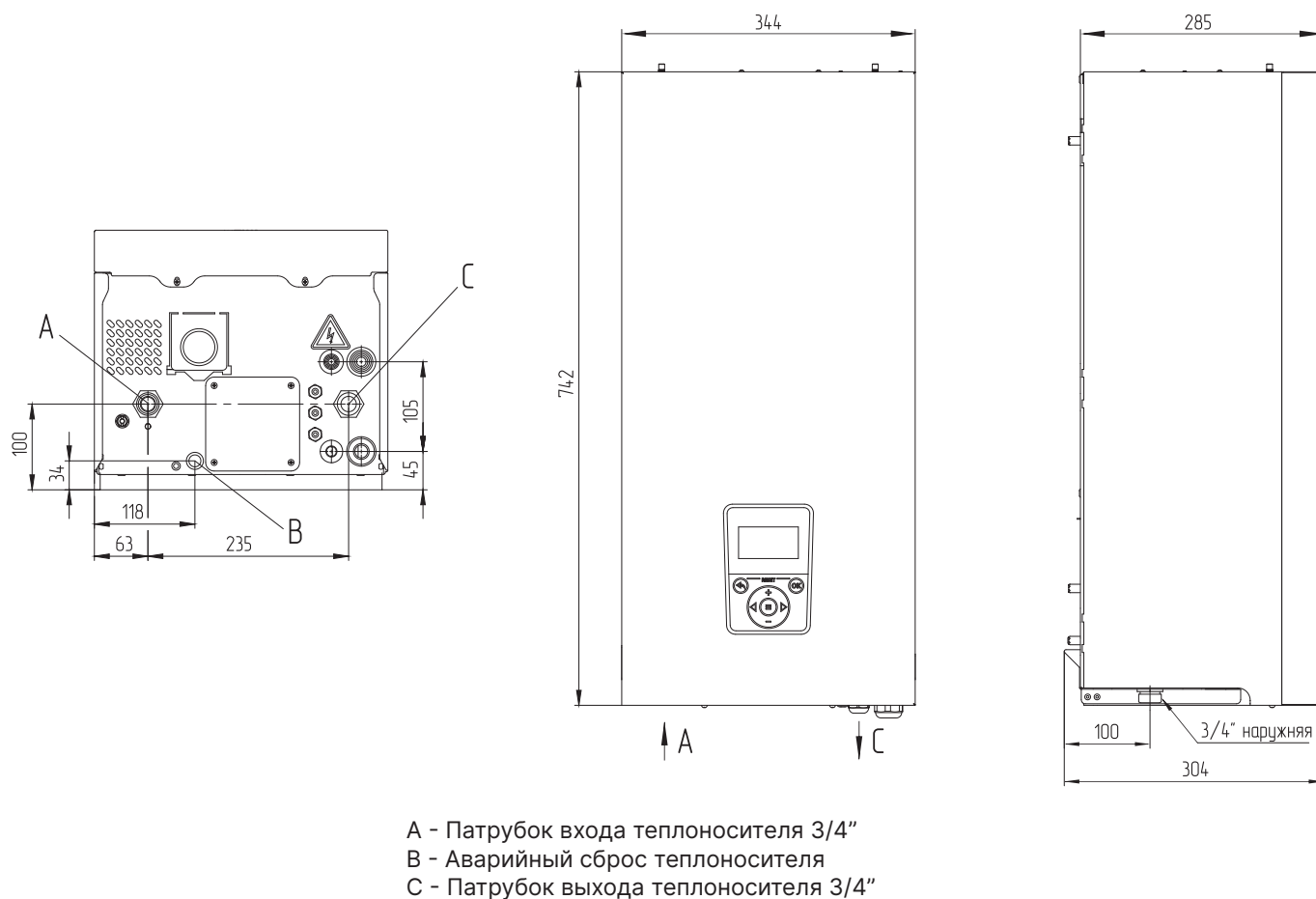
Рис. 6 Габаритные размеры ZOTA MK-X Slim и ZOTA MK-X Slim Grey 6-24 кВт
