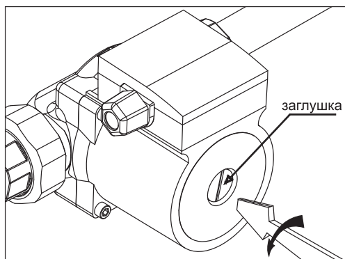
Рис. 5 Удаление воздуха из насоса
