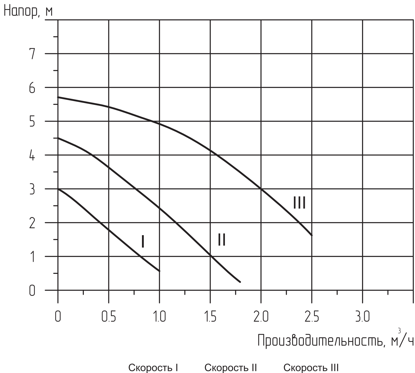
Рис. 1 Остаточный напор для циркуляционного насоса 15-6S (для котлов ZOTA MK-X Slim и ZOTA MK-X Slim Grey 6-24 кВт)
