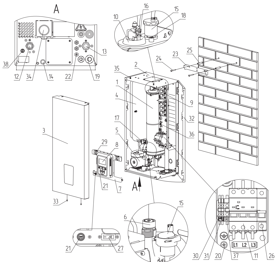
Рис. 2 Устройство котла ZOTA MK-X Slim и ZOTA MK-X Slim Grey 6-24 кВт
