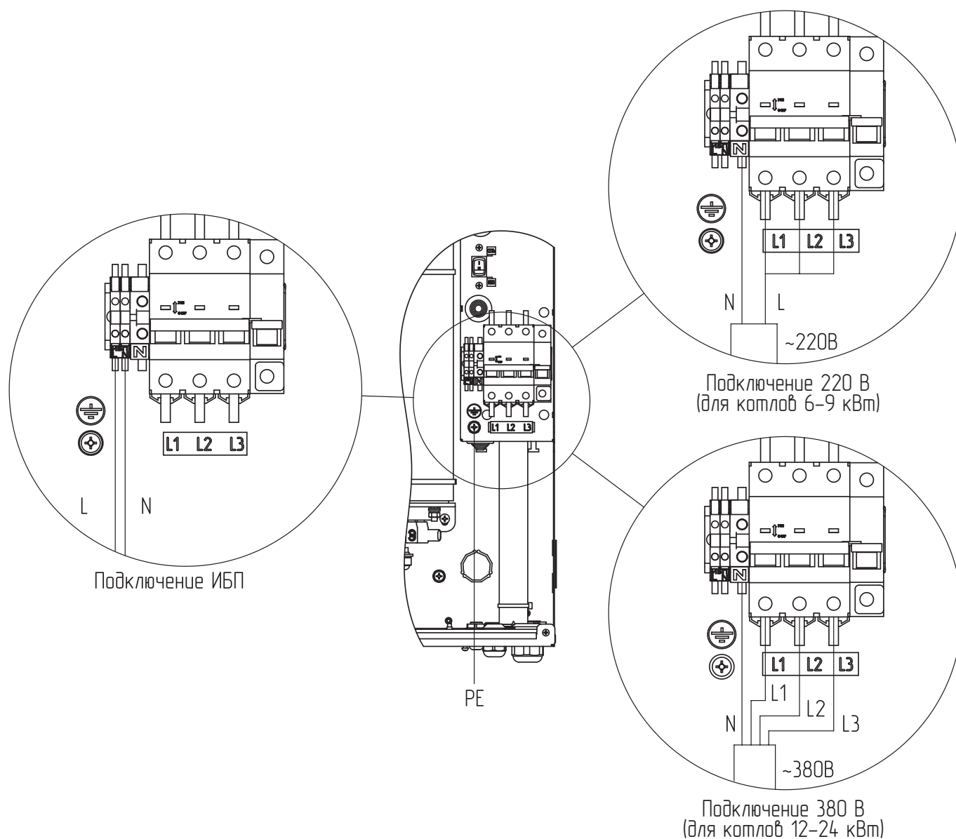
Рис. 3 Схема подключения котла ZOTA МК-X Slim и ZOTA МК-X Slim Grey 6-24 кВт
