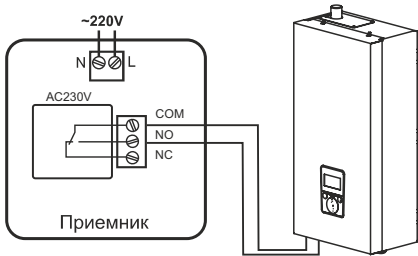
Беспроводной термостат
