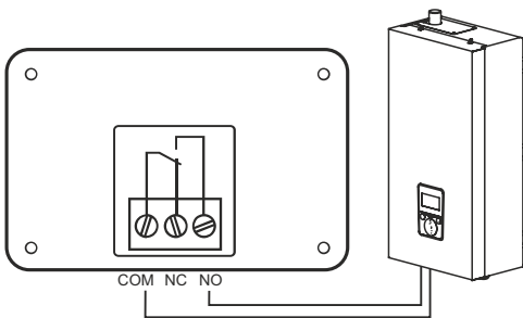
Проводной термостат
