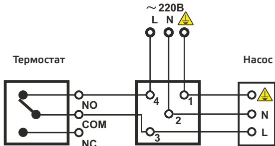
Схема подключения внешнего комнатного термостата к циркуляционному насосу
