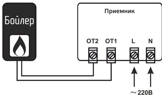
Схема подключения приемника терморегулятора ZOTA ZT-84W Wi-Fi OT+
