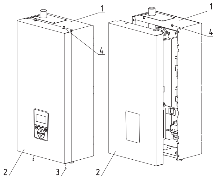
Рис. 14 Снятие кожуха
