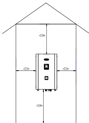
Рис.4 Схема установки миникотельной
