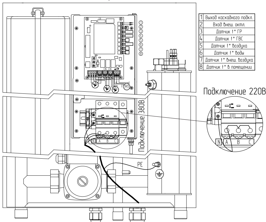
Рис.3 Схема подключения миникотельной
