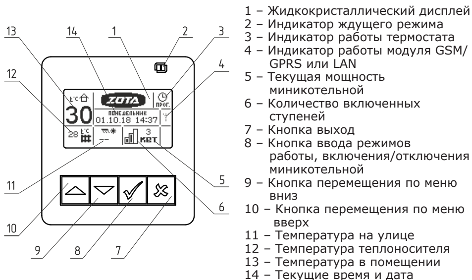
Рис. 2 Расположение органов управления и индикации на передней панели
