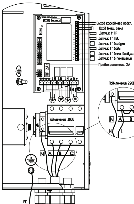
Рис. 3 Схема подключения электроводонагревателя
