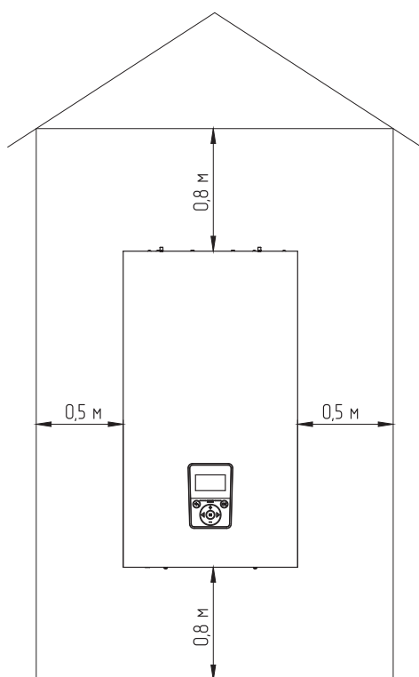
Рис. 7 Схема размещения котла в котельной
