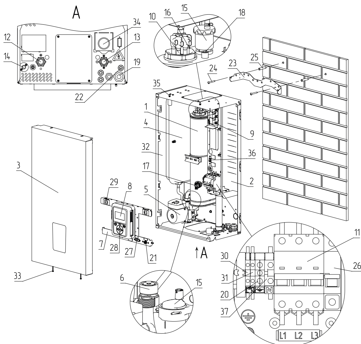
Рис. 3 Устройство электрического котла ZOTA МК-X V2 от 4,5 до 24 кВт
