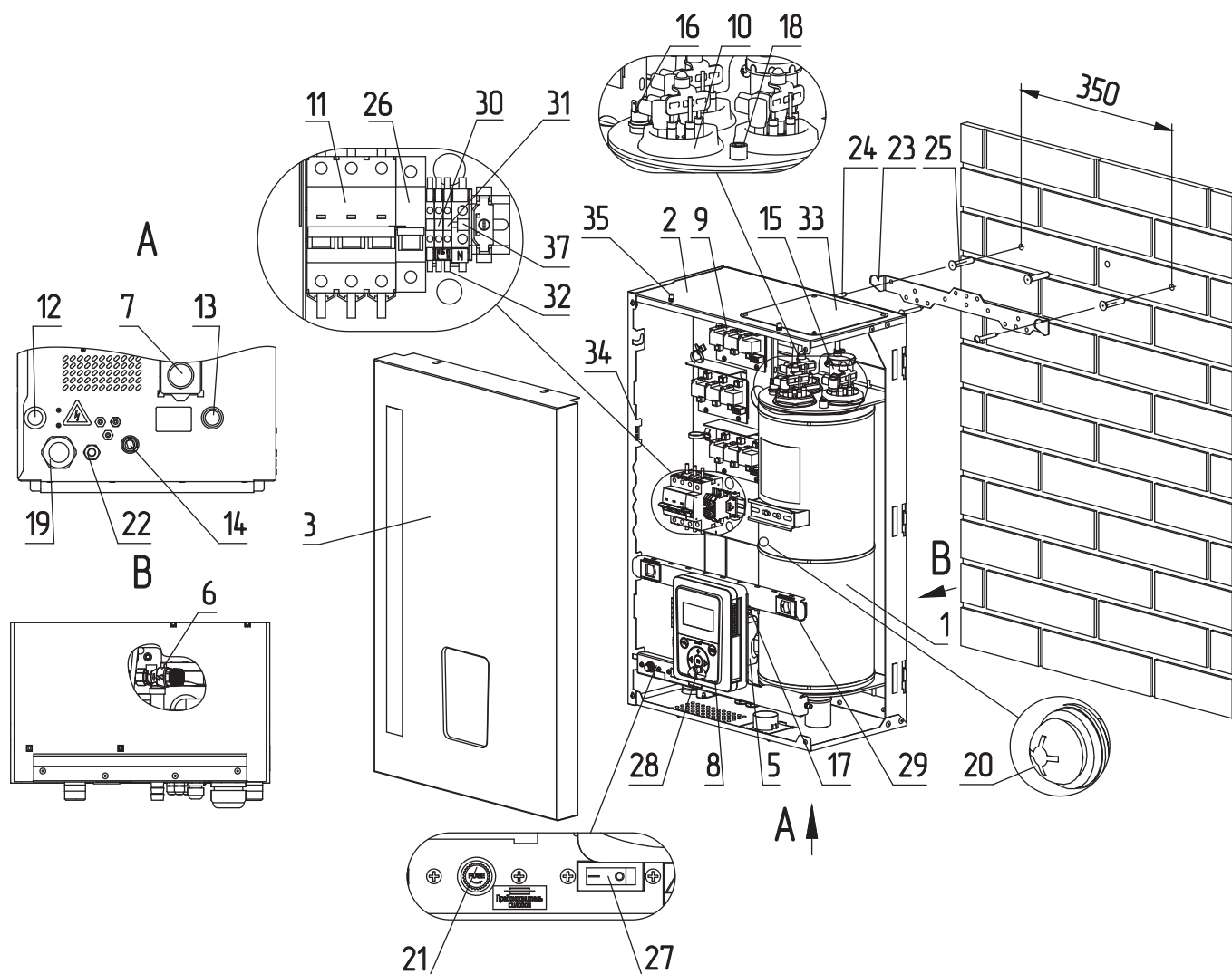
Рис. 4 Устройство электрического котла ZOTA МК-Х от 30 до 36 кВт
