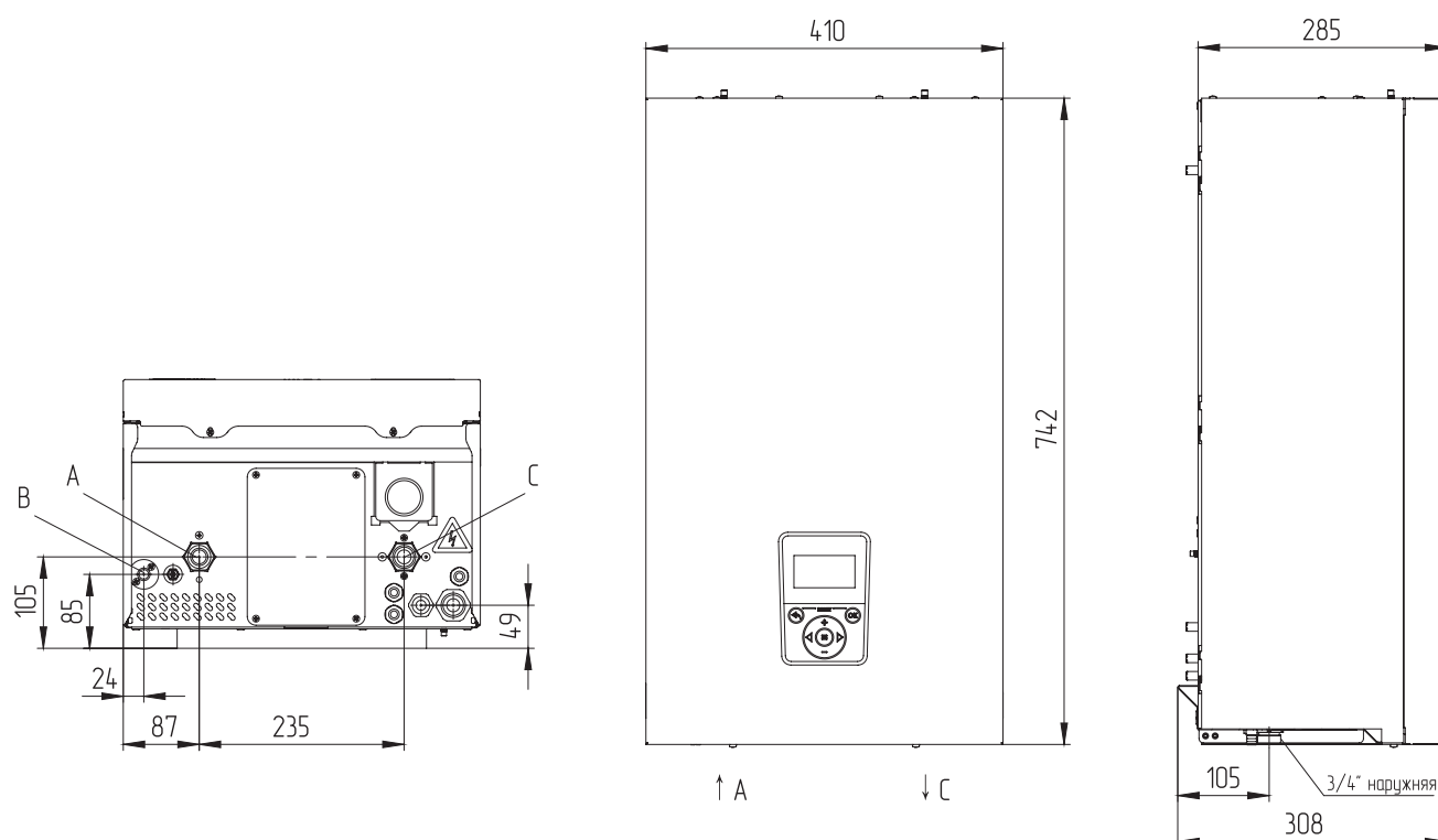
Рис. 9 Габаритные размеры ZOTA MK-X V2 от 4,5 до 24 кВт
