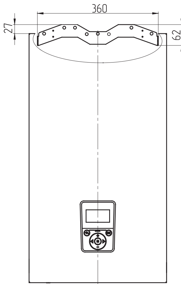
Рис. 11 Позиционирование котла относительно кронштейна
