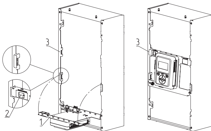
Рис. 13 Откидывание и сервисное положение кронштейна
