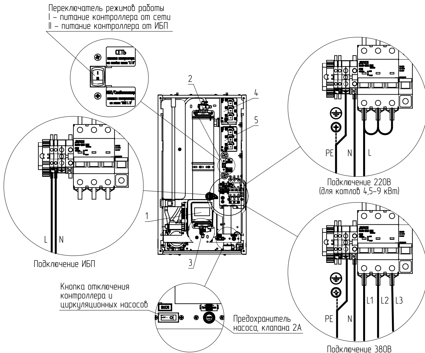
Рис. 5 Схема подключения и органы управления электрического котла ZOTA MK-X V2 от 4,5 до 24 кВт
