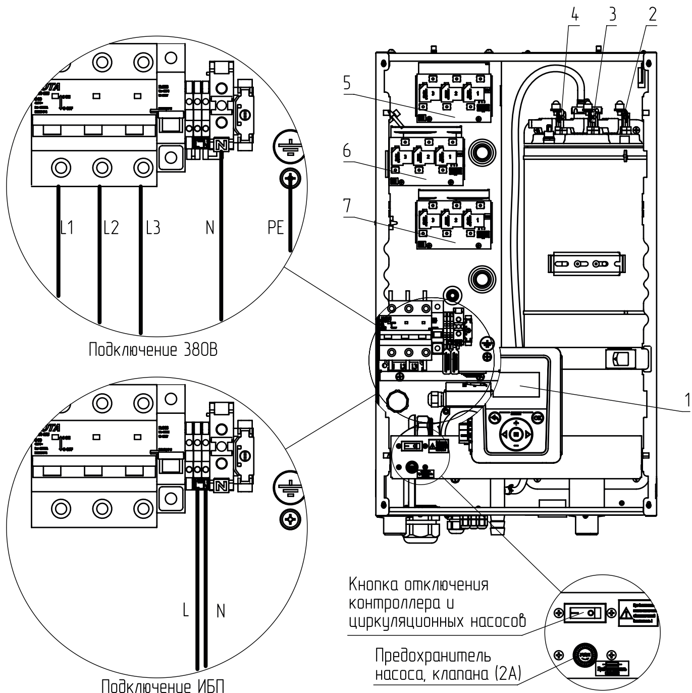
Рис. 6 Схема подключения и органы управления электрического котла ZOTA МК-Х от 30 до 36 кВт
