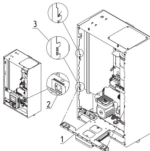
Рис. 13 Откидывание кронштейна
