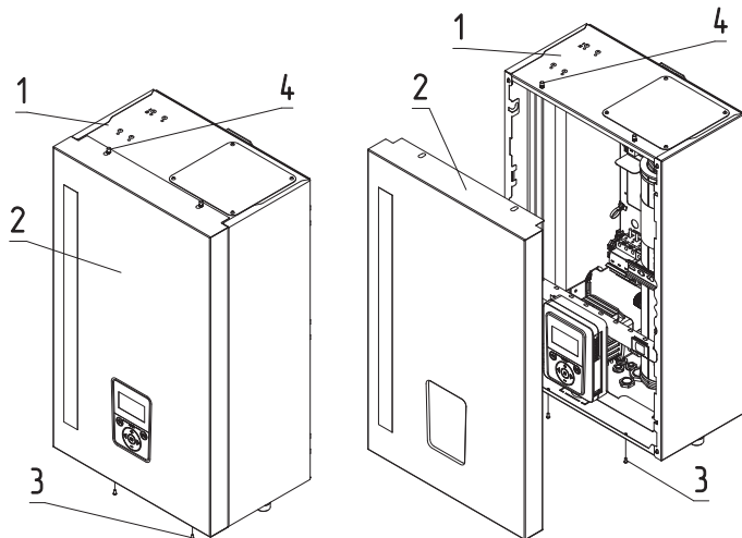
Рис. 12 Снятие кожуха
