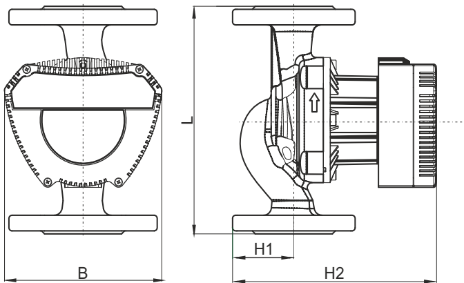
Монтажные размеры насосов с фланцевым соединением
