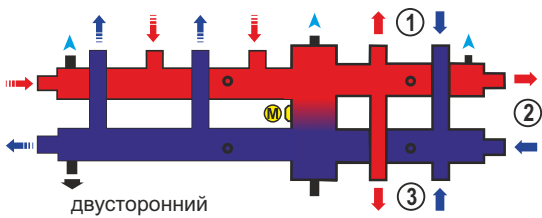
3 контура GR4930000029
