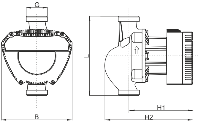
Монтажные размеры насосов с резьбовым соединением
