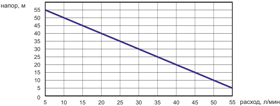
Расходно-напорные характеристики центробежных насосов LOTOS
