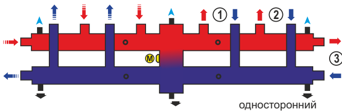
3 контура GR4930000030
