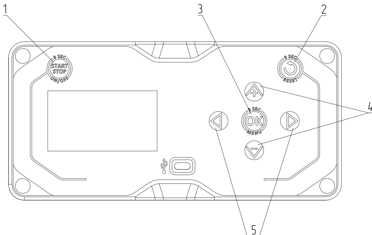
Рис. 11 Функциональные клавиши контроллеров ZOTA серии C-Line 200SFA
