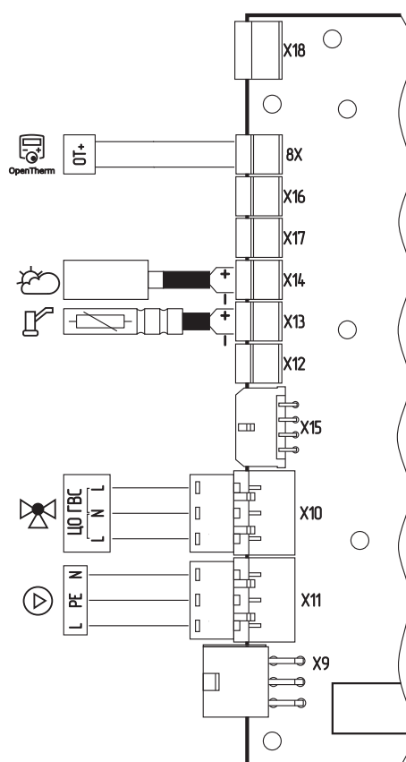
Рис.11 Подключение клапана приоритета бойлера ГВС, датчиков ГВС и улицы, и устройства OpenTherm к контроллеру «ZOTA X-Line 100E»
