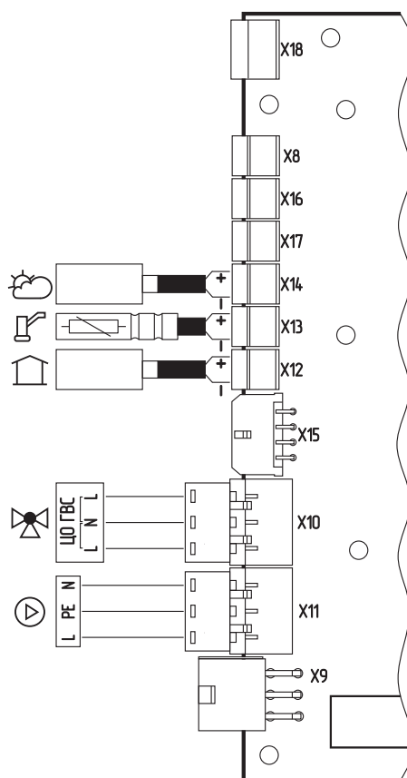
Рис.10 Подключение клапана приоритета бойлера ГВС, датчиков температуры в помещении, ГВС и улицы к контроллеру «ZOTA X-Line 100E»
