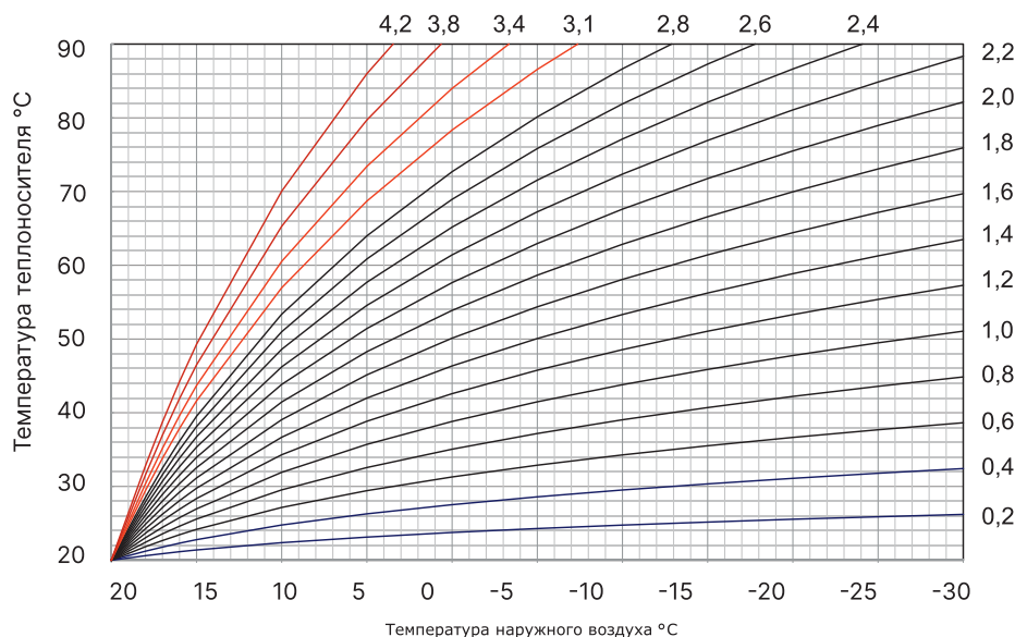
Рис.7 Выбор коэффициента «кривой» погодозависимого регулирования
