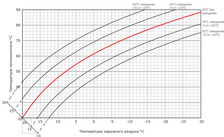
Рис.8 Смещение коэффициента кривой погодозависимого управления (на примере кривой 2).
