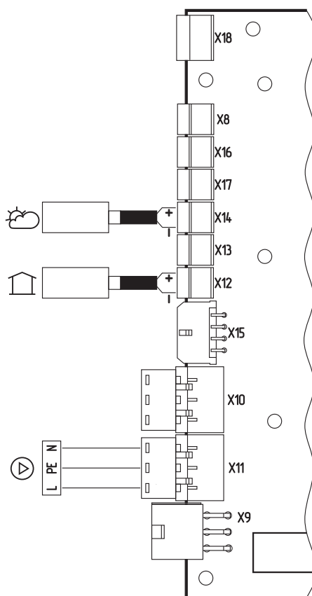
Рис.9 Подключение датчиков температуры в помещении и улицы к контроллеру «ZOTA X-Line 100E»
