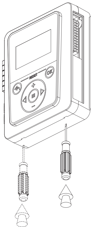
Рис.12 Демонтаж лицевой панели
