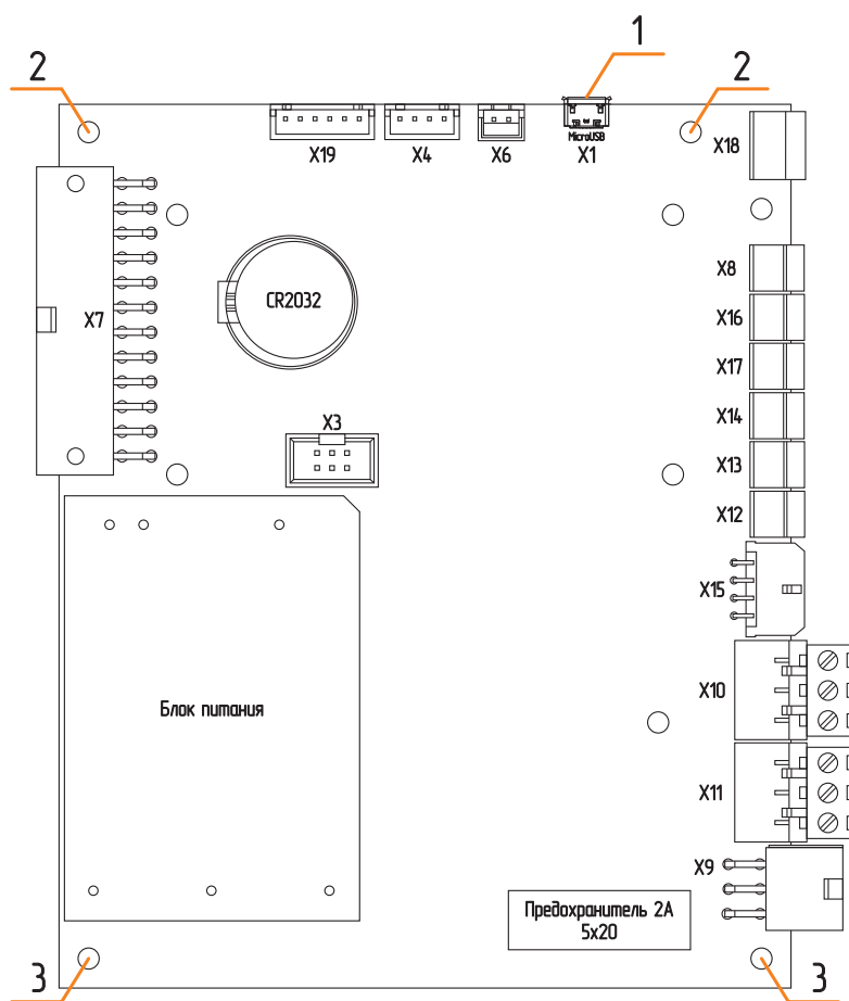
Рис.13 Плата контроллера
