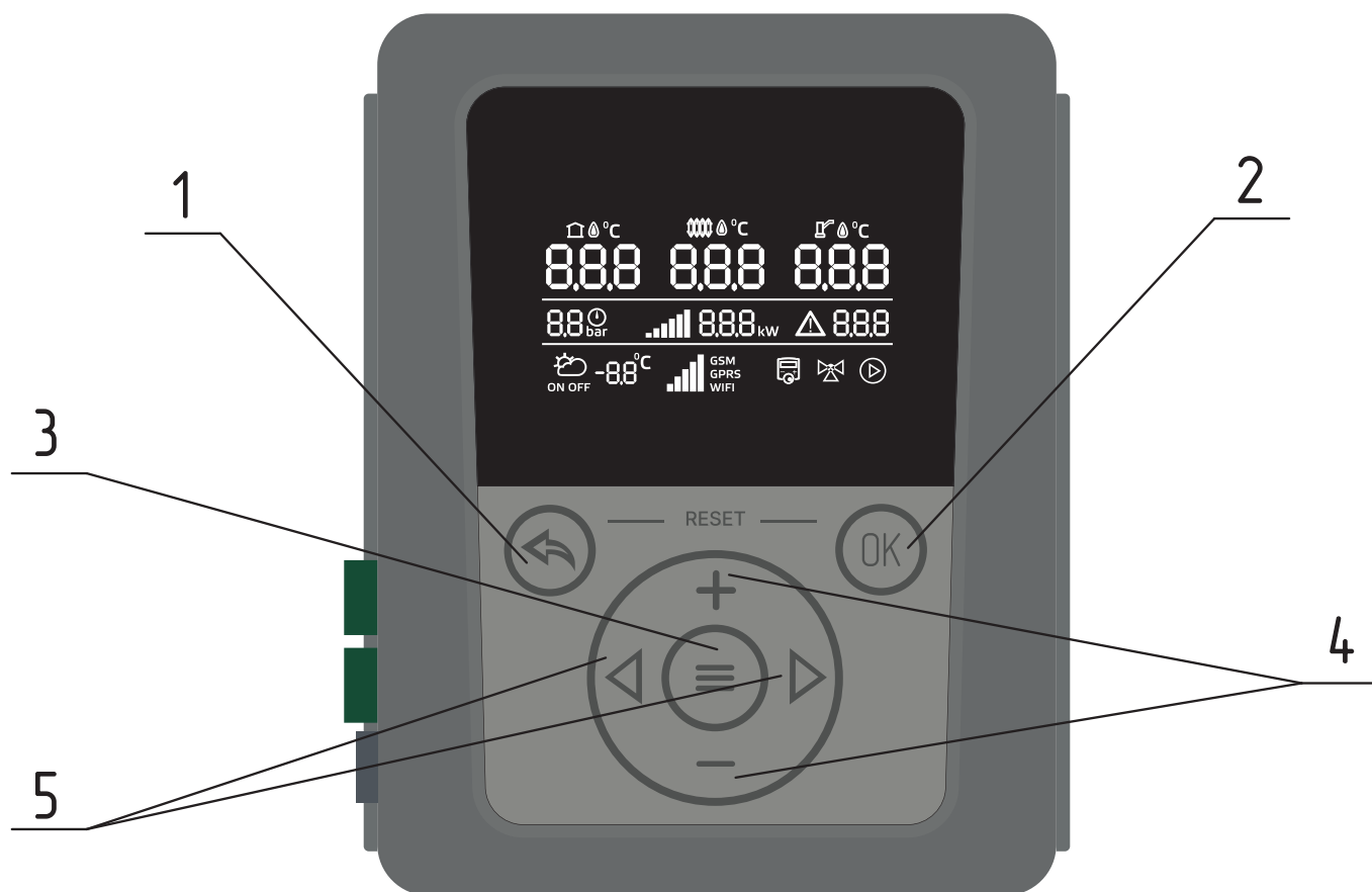
Рис.5 Внешний вид контроллера «ZOTA X-line 100E»
