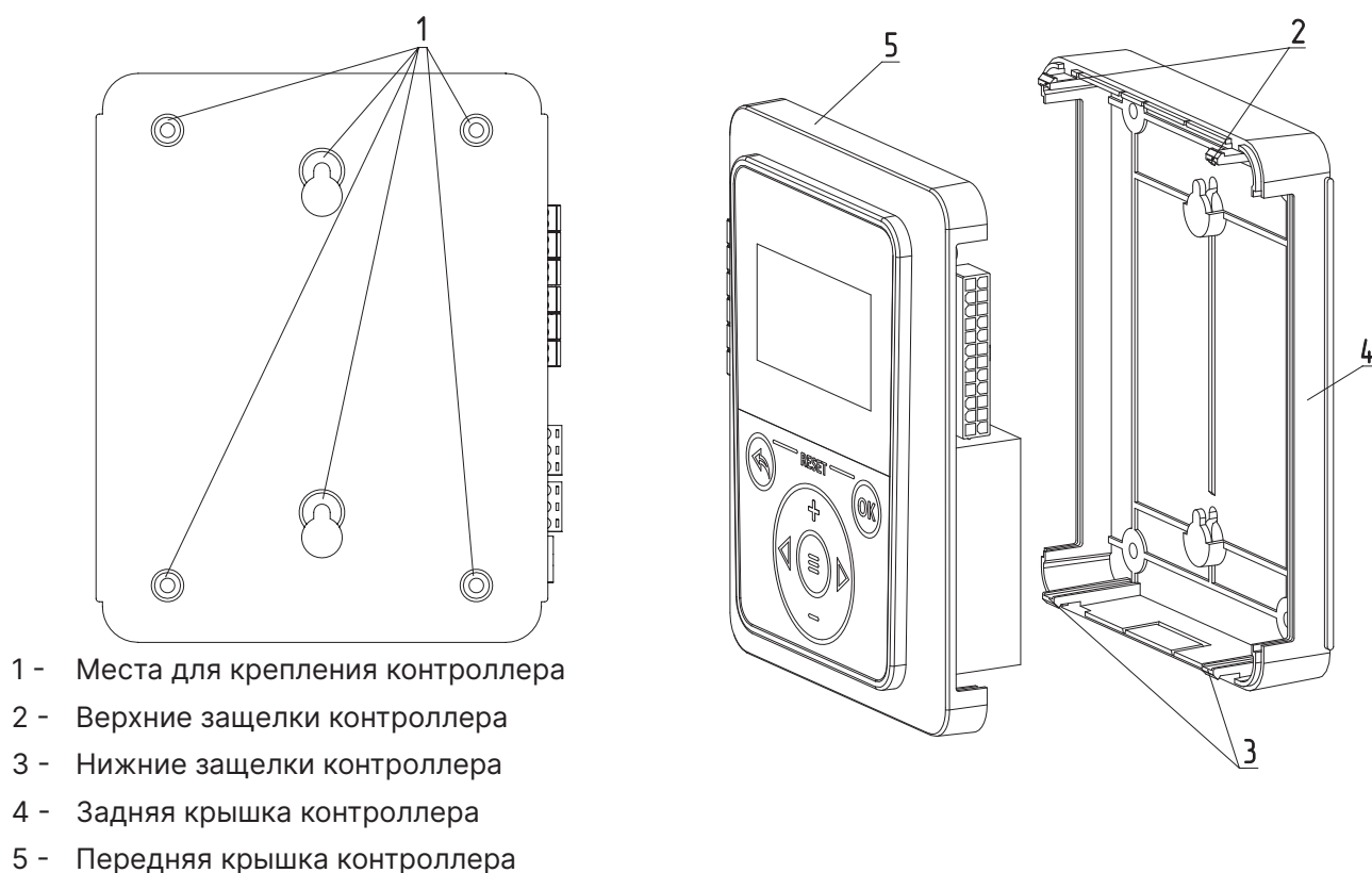
Рис.1 Корпус контроллера «ZOTA X-Line 100E»
