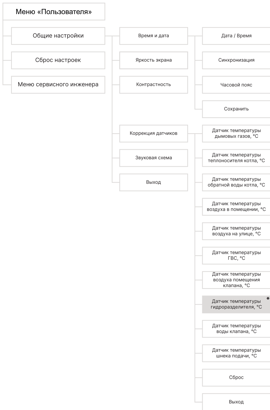
Рис.20 Блок-схема меню пользователя (продолжение)
