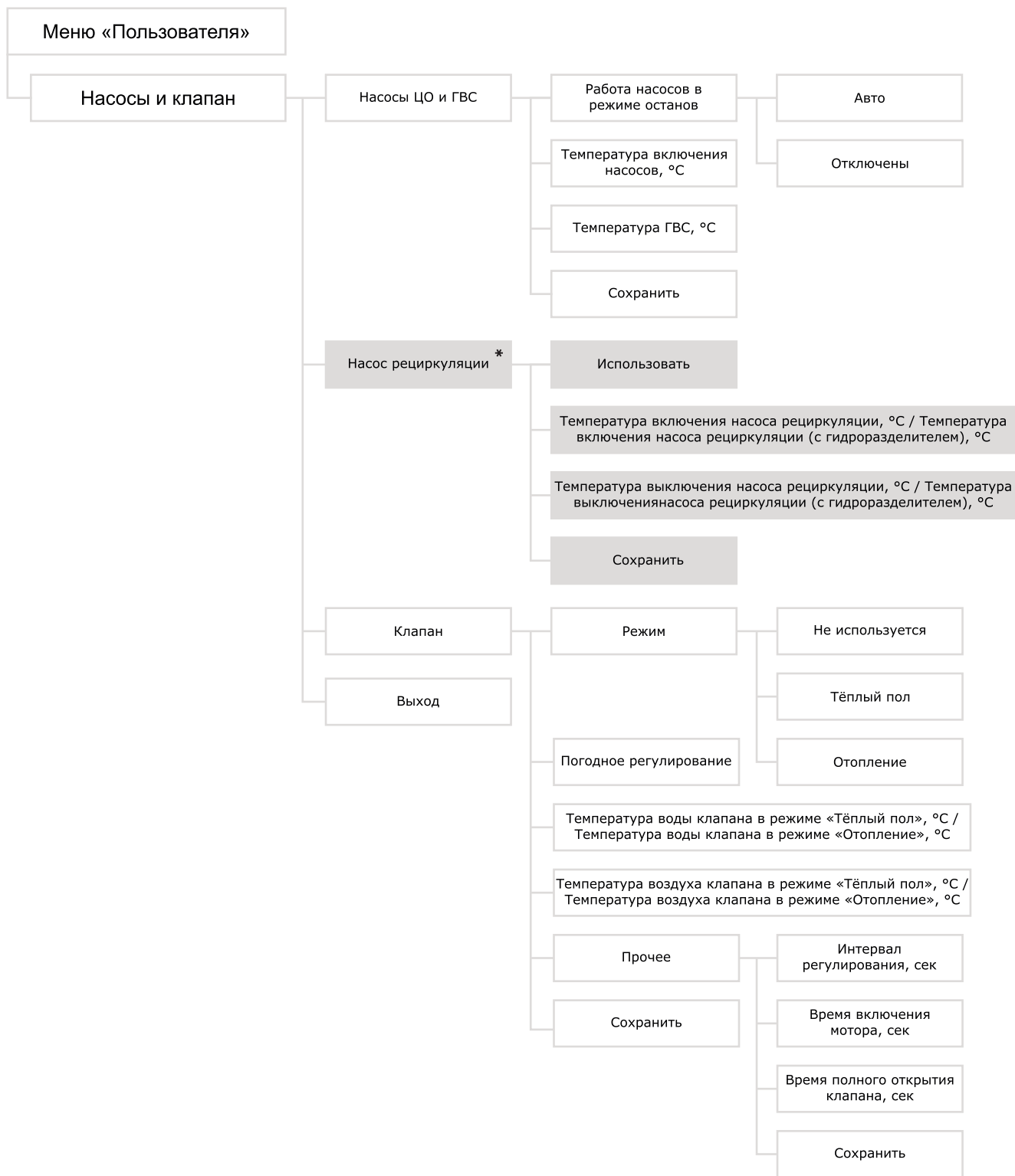
Рис.17 Блок-схема меню пользователя (продолжение)
