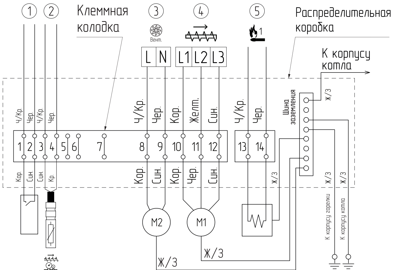
Рис.6 Схема распределительной коробки контроллеров ZOTA серии I-Line 223SFA для котлов ZOTA Stahanov 16-65 кВт
