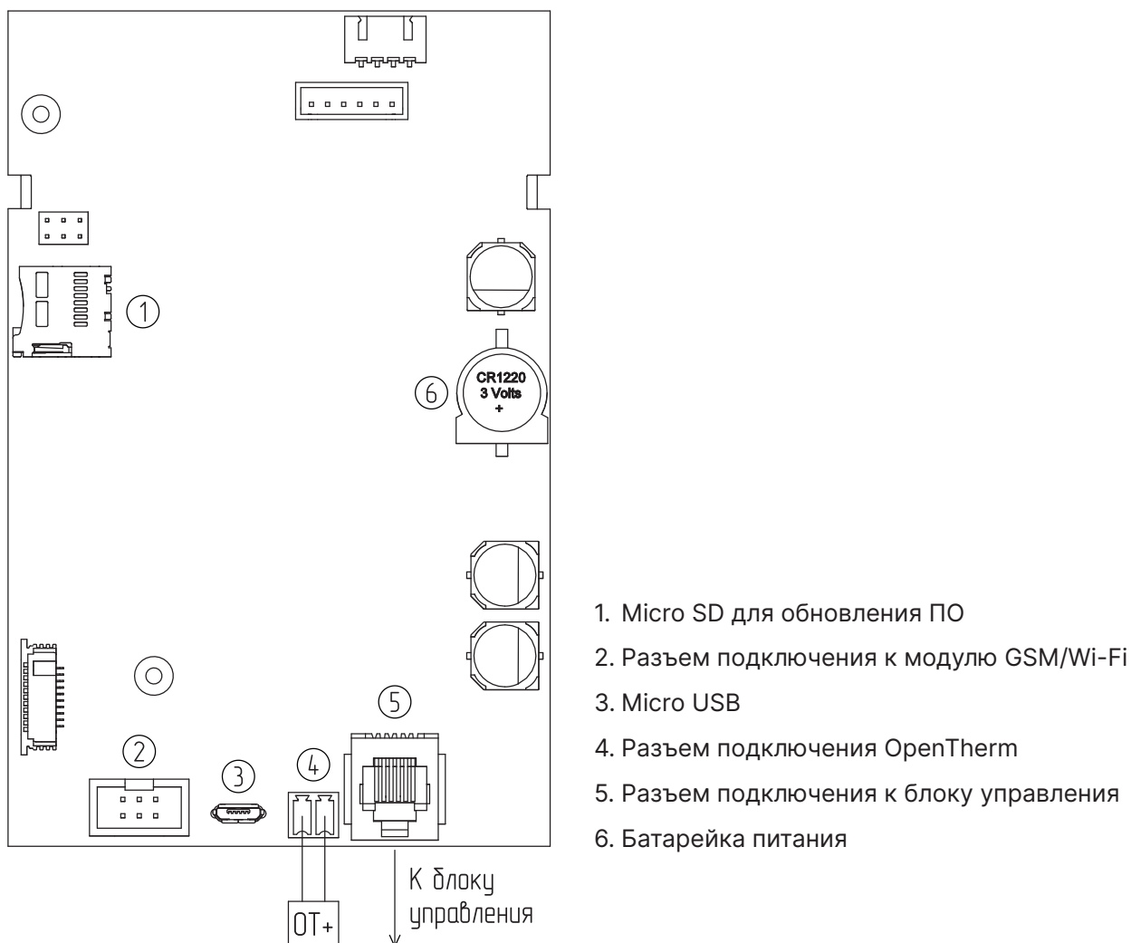
Рис.10 Схема платы блока индикации контроллеров ZOTA серии R-Line и серии I-Line
