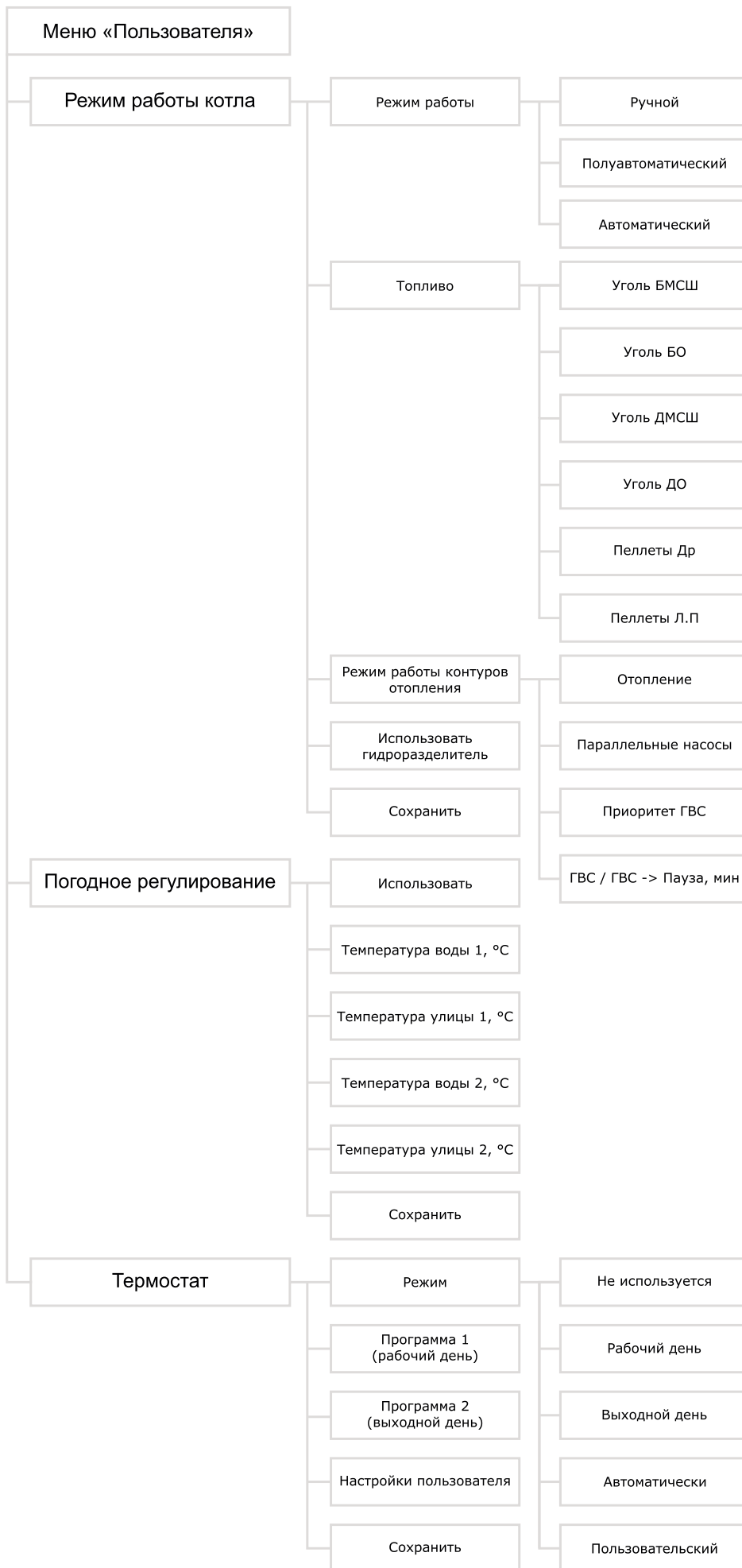
Рис.16 Блок-схема меню пользователя (продолжение)
