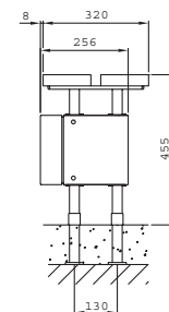
4-трубная модель
