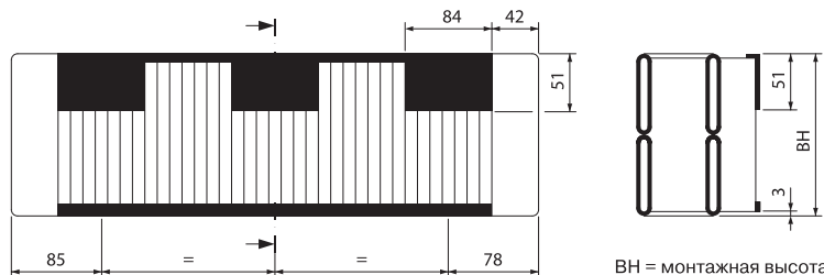
BH = монтажная высота
