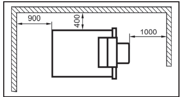
Рис.: Минимальный отступ от стены
