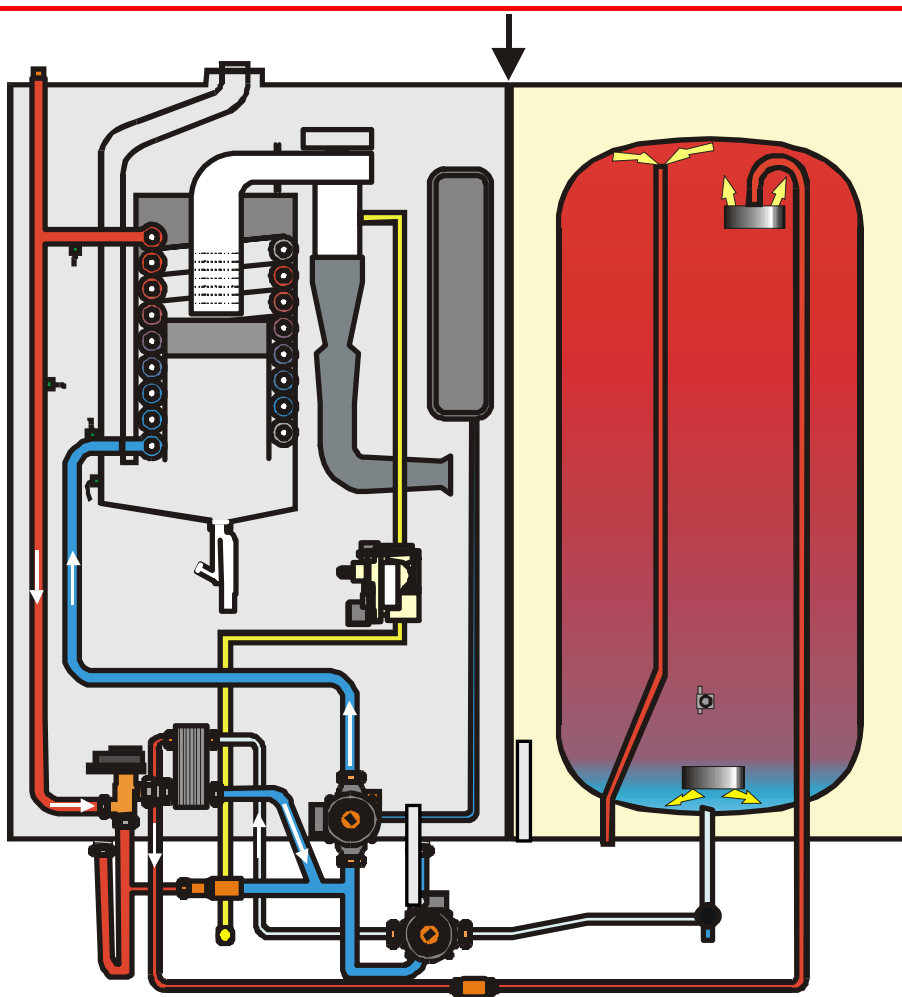
Газовый конденсационный настенный котел CGW
