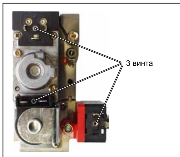
Рис.: Газовый комбинированный клапан
