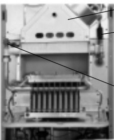
Сборник отходящих газов Датчик температуры в обратной линии Защитный ограничитель температуры
