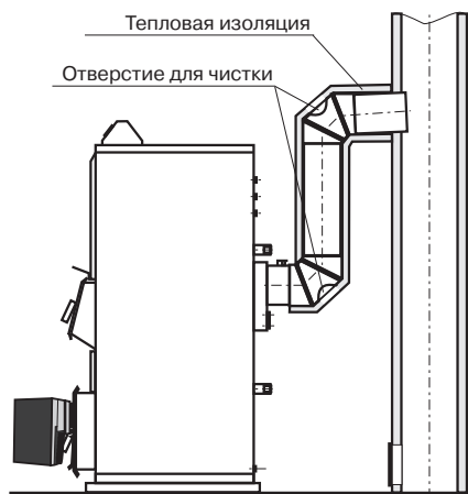
Способ подключения котла ЕКО-СКВ к дымовой трубе (при работе с наддувной горелкой)
