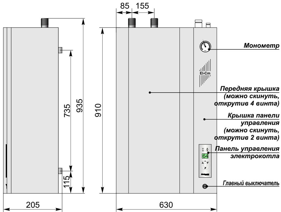
Рис 1. - Основные размеры электрокотла EI-Cm
