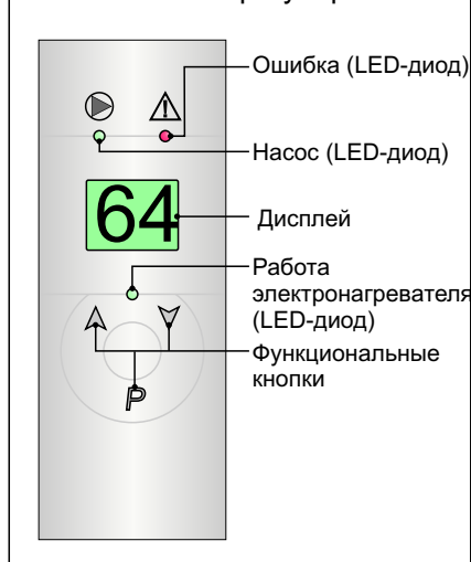
Рис 5. - Панель регулировки
