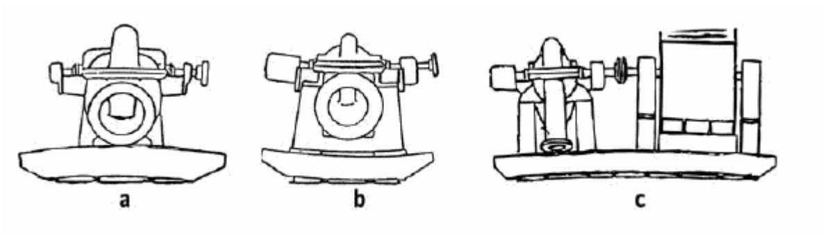
Рисунок 4. Примеры повреждения/деформации фундаментов
