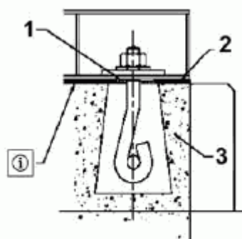
Рисунок 5. Фундаментный болт
