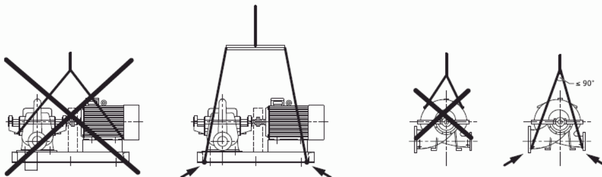
Рисунок 1. Обращение с насосом при погрузке и транспортировке
