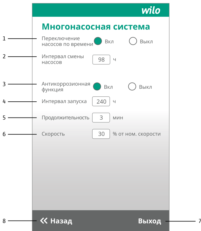
Рис. 5.1.12. Настройка системы из нескольких насосов
