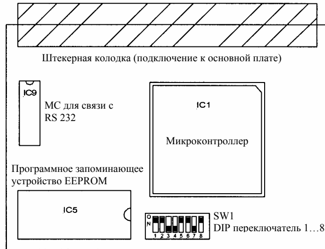
Рис. 4: Плата микроконтроллера
