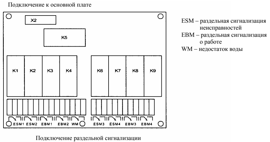
Рис. 6: Плата раздельной сигнализации и работы каждого насоса
