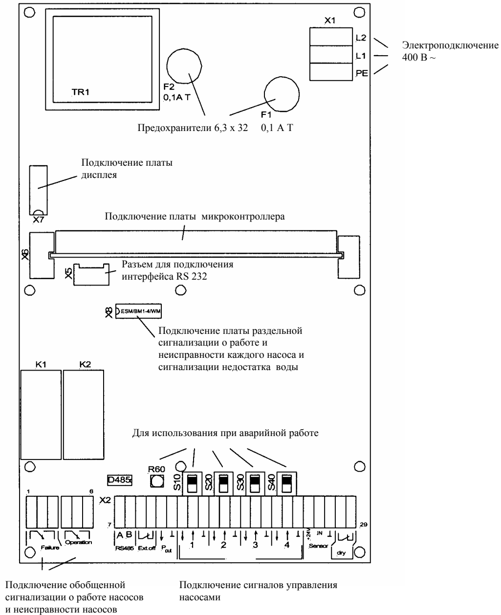
Рис. 3: Основная плата
