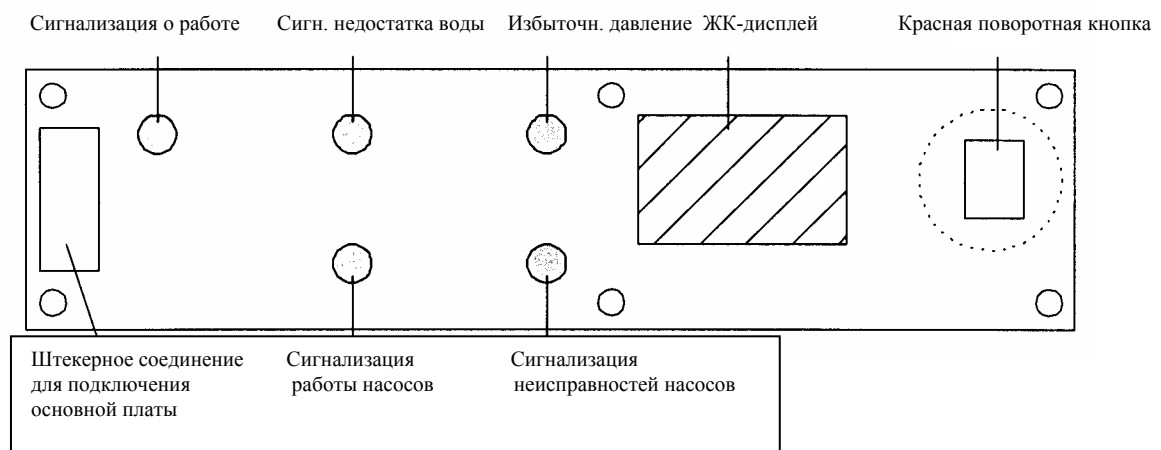
Рис. 5: Плата дисплея
