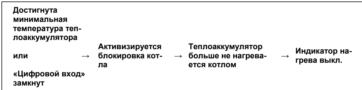
Рис.6.2 Блокировка нагрева
