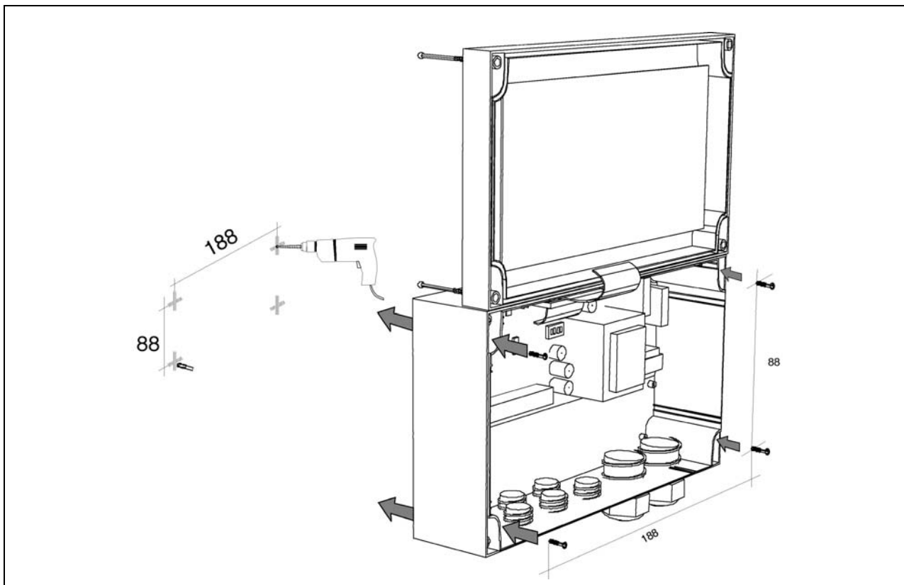
Рис.4.1. Монтаж корпуса
