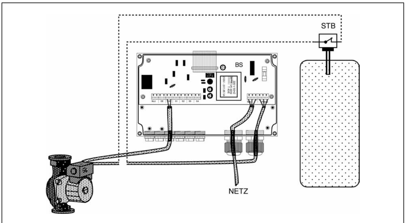
Рис.6.3. Система с предохранителем по температуре
