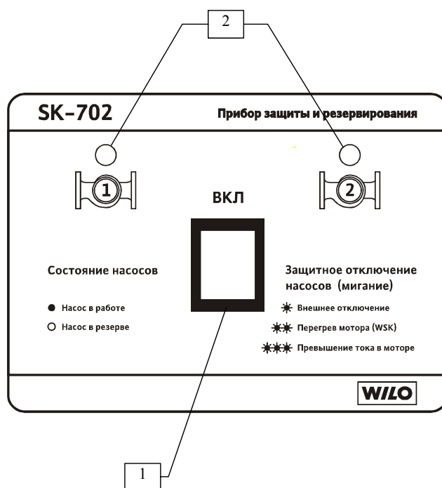
Рис. 1 Лицевая панель прибора
