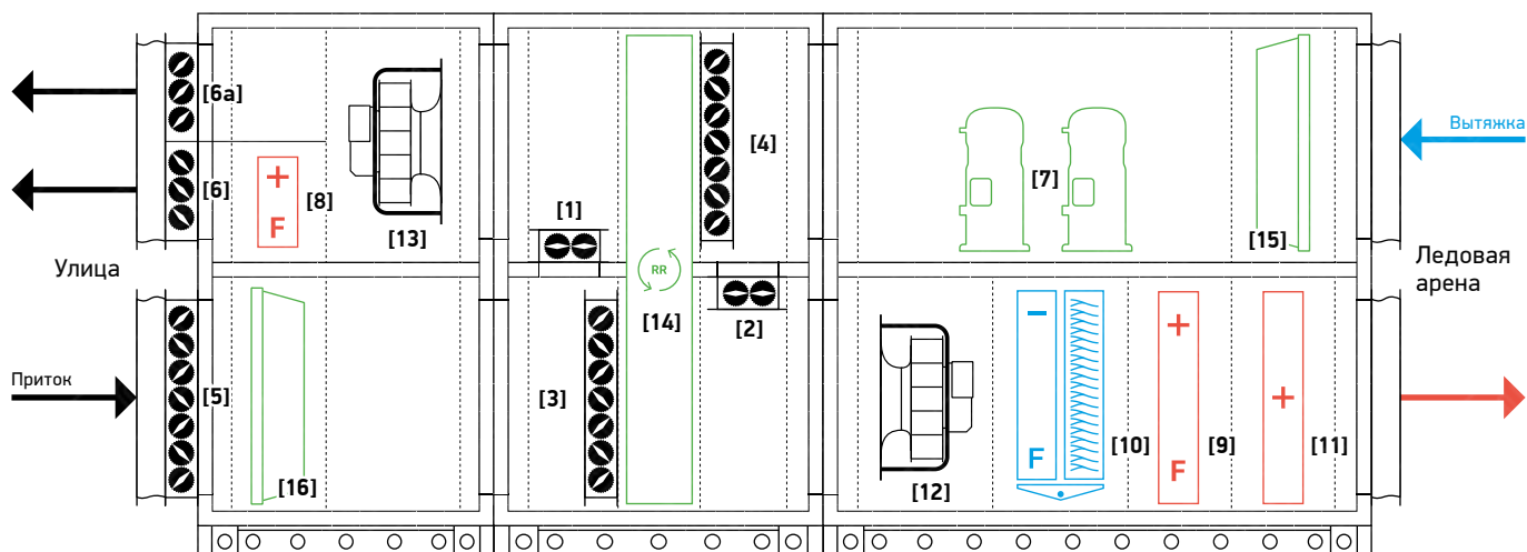
Рис. 38. Принципиальная схема установки WHEEL SIRIUS ICE
