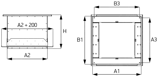
Схема 84. Монтажный стакан /TSN.N4
