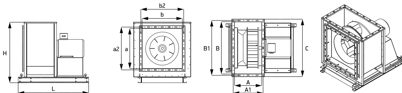
Схема 63. Габаритные и присоединительные характеристики вентиляторов WHEEL SHAULA FAN /FPL (выхлоп влево, 90°)
