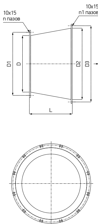
Схема 116. Диффузор на выхлопе
