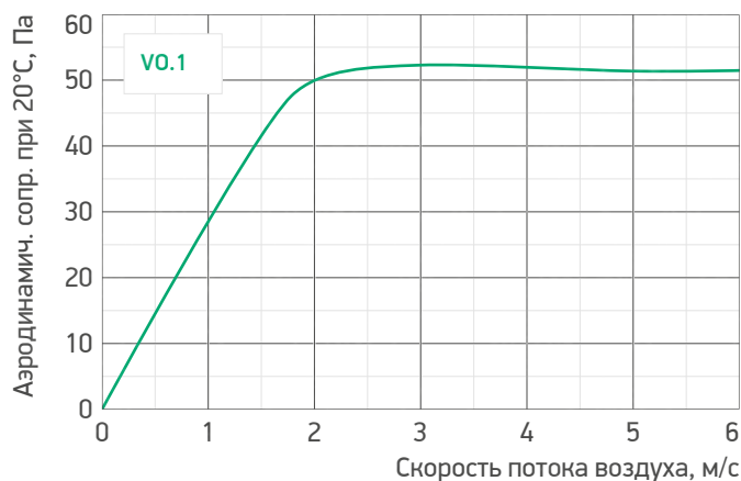
Гр. 34. Аэродинамические характеристики обратных клапанов /VO.1
