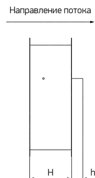
Схема 119. Клапан обратный вертикальный для работы на вытяжку VO.1, VOK.1, VOD.1
