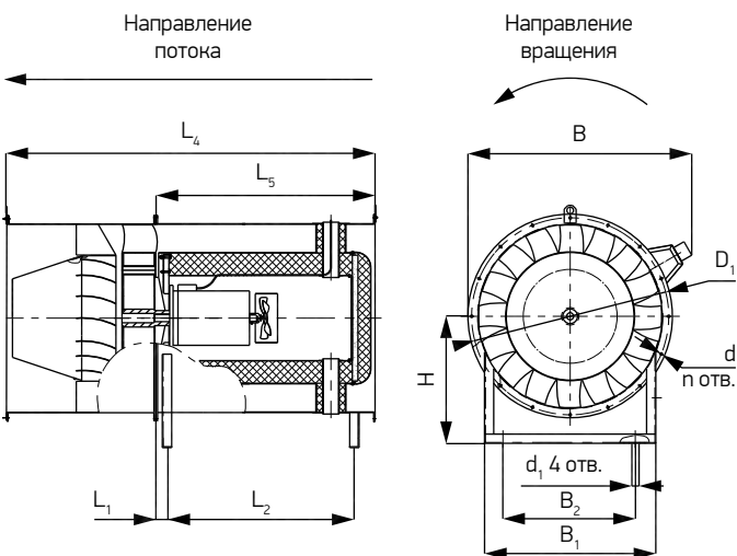
Схема 112. Исполнение SE.400_ F.SA
