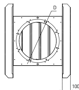
Схема 131. Стакан монтажный с обратным клапаном приток для плоской кровли TSA.C_, TSC.C_, TSE.C_
