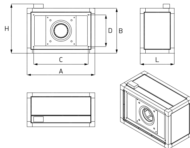
Рис. 4. Габаритные и присоединительные размеры вентиляторов /FECI
