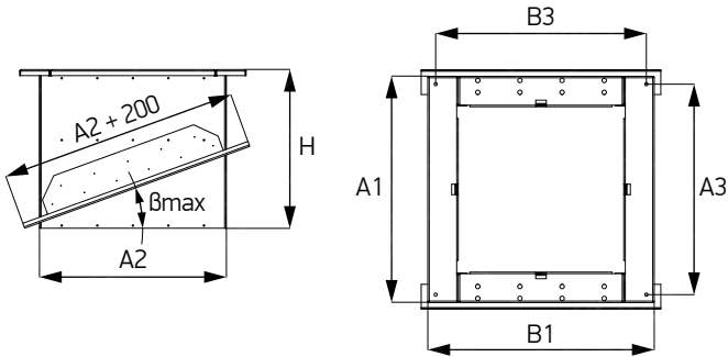
Схема 83. Монтажный стакан /TSN.N2
