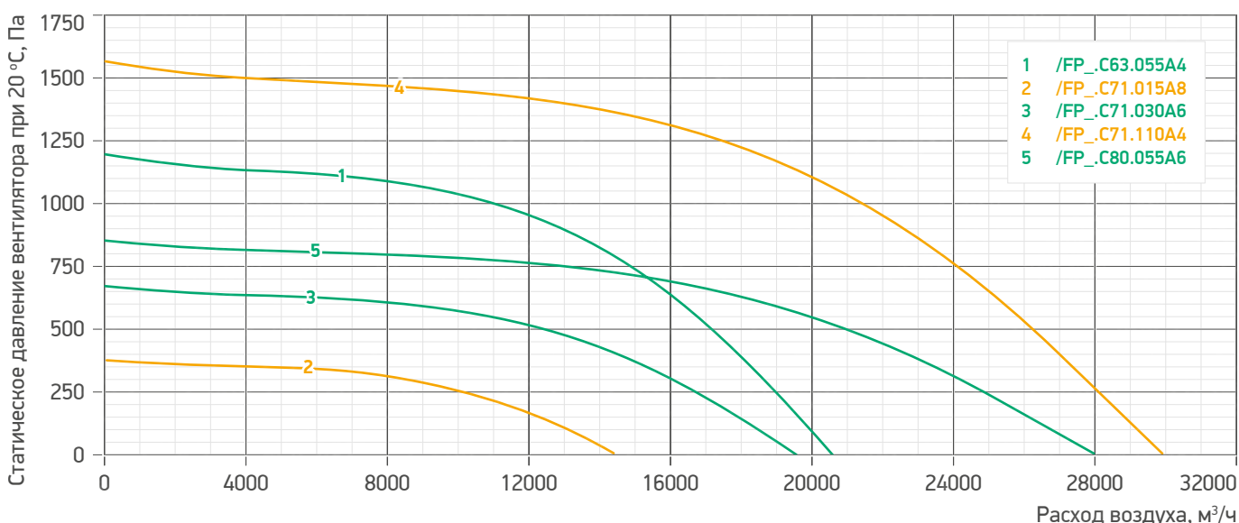
Гр. 36. Аэродинамические характеристики вентиляторов WHEEL SHAULA ROOF /FP_ (продолжение)
