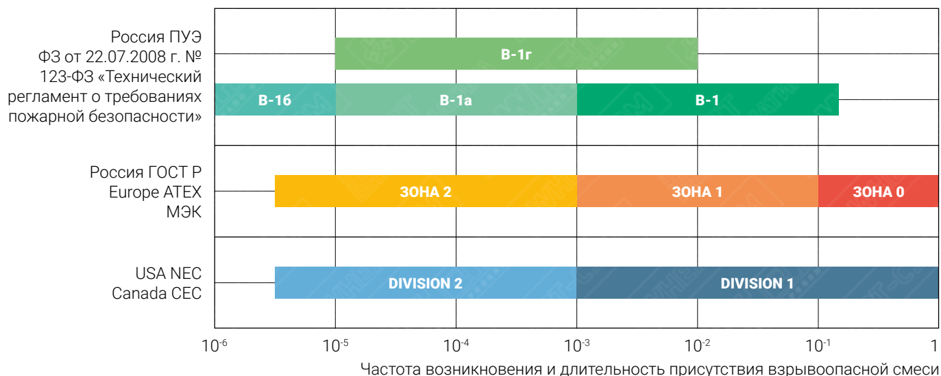
Рис. 151. Возрастание потенциальной опасности взрыва
