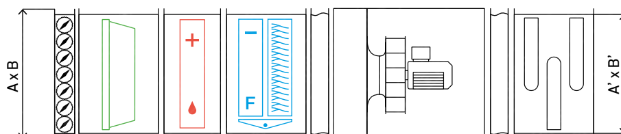
Схема 1. Габаритные и присоединительные характеристики установок WHEEL WEGA XP
