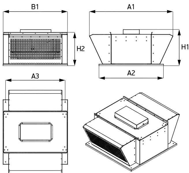
Табл. 51. Габаритно-весовые характеристики вентиляторов WHEIL SHAULA ROOF /FB
