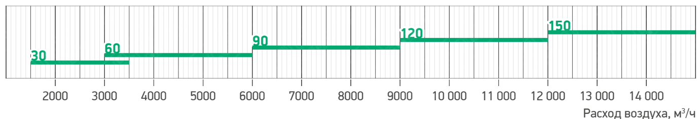
Гр. 71. Рекомендуемые типоразмеры установок WHEEL SIRIUS TOP в зависимости от расхода воздуха
