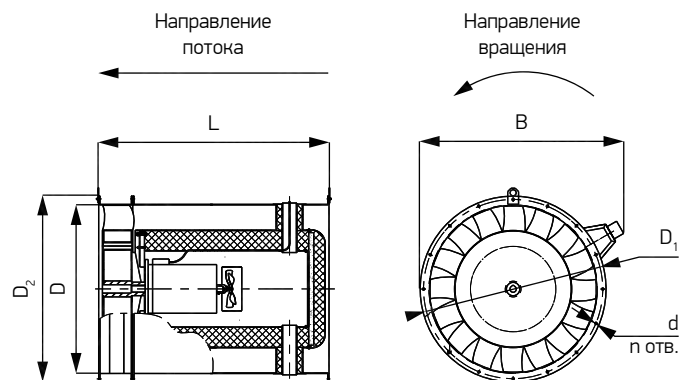
Табл. 123. Габаритные характеристики вентиляторов /FA.R16
