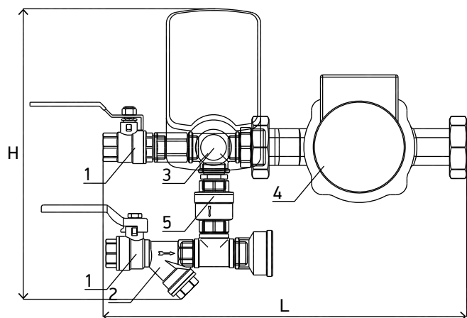
Схема 158. Смесительный узел /MUB...
