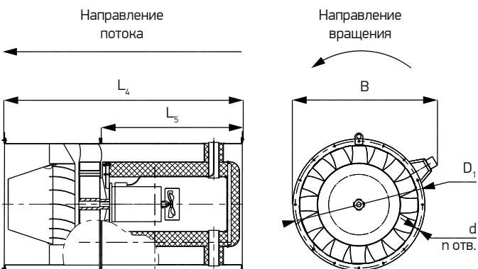
Схема 112. Исполнение SE.400_ F.SA
