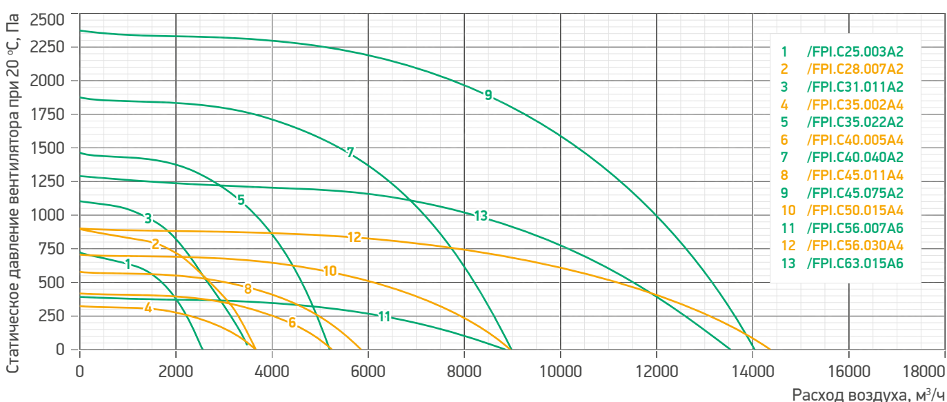
Гр. 17. Аэродинамические характеристики вентиляторов WHEEL SHAULA BOX /FPI (продолжение)
