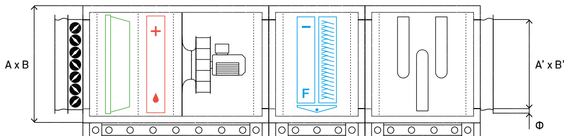
Схема 66. Габаритные размеры установок WHEEL POLARIS
