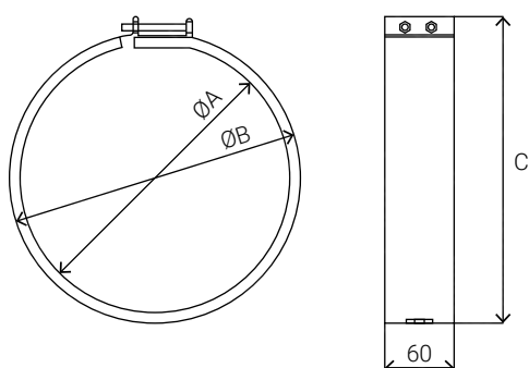
Схема 43. Габаритные размеры хомутов быстросъемных /Г.1
