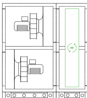
Схема 71. 2% (переток вытяжного воздуха в приточный, перетекание воздуха оставшегося в каналах регенератора)
