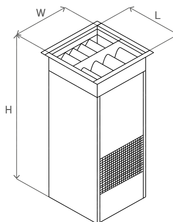
Схема 80. Габаритные размеры внутреннего модуля установок WHEEL POLARIS TOP
