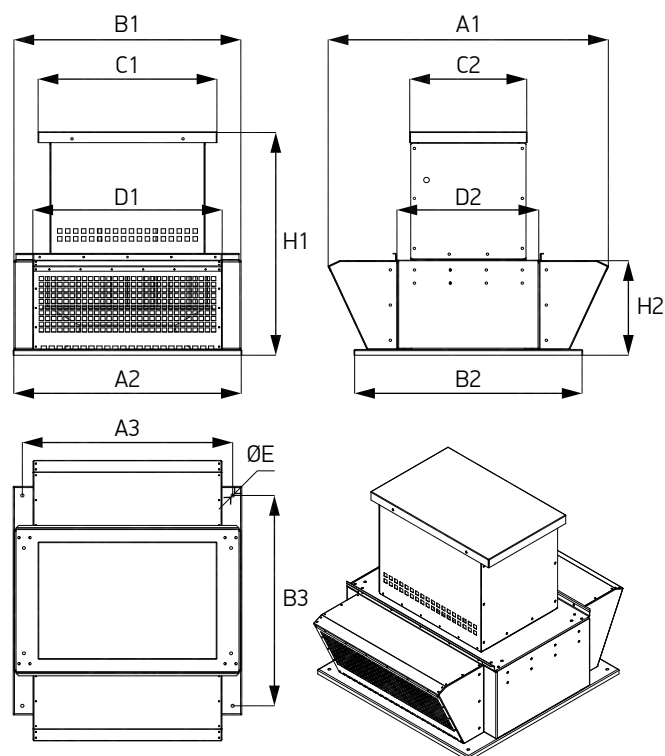
Схема 81. Исполнение с выхлопом в стороны WHEEL SHAULA ROOF SE /FPH
