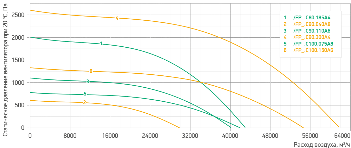
Гр. 38. Аэродинамические характеристики вентиляторов WHEEL SHAULA ROOF /FB_
