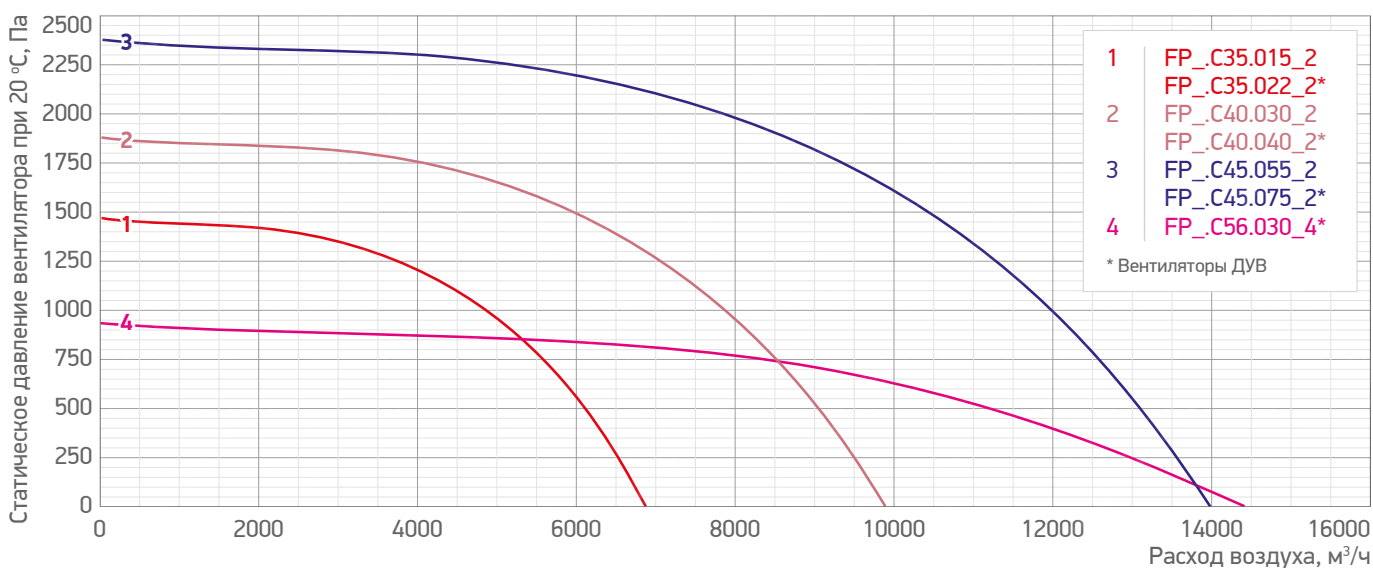
Табл. 60. Электрические характеристики вентиляторов WHEEL SHAULA FAN /FP_ (расход до 14 000 м³/ч)
