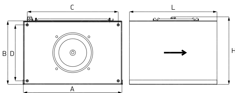
Схема 2. Габаритные и присоединительные размеры вентиляторов /FR
