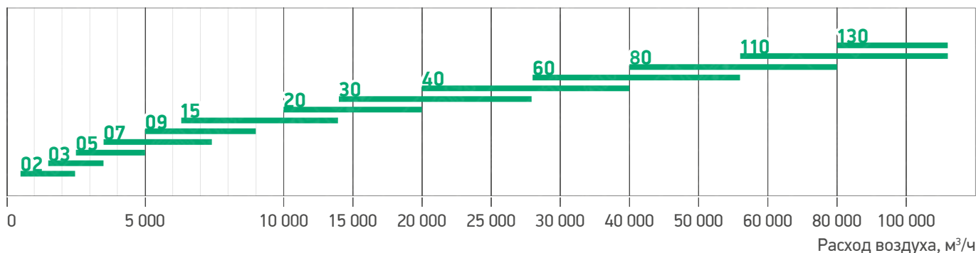
Гр. 43. Рекомендуемые типоразмеры в зависимости от расхода воздуха установок WHEEL SIRIUS
