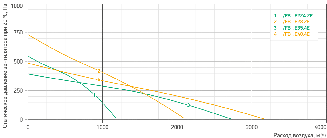
Гр. 39. Аэродинамические характеристики вентиляторов WHEEL SHAULA ROOF /FB_ (продолжение)
