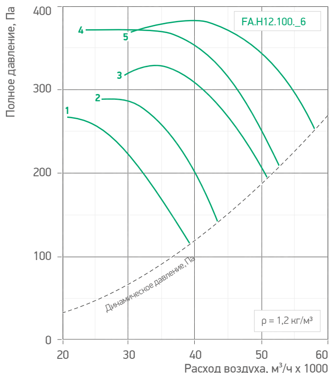
Гр. 102. Аэродинамические характеристики вентилятора /FA.H12.100_А6
