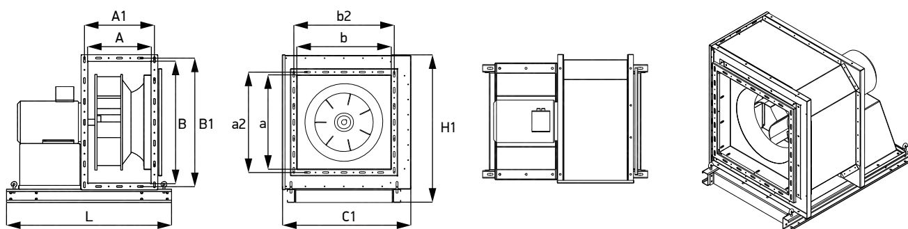
Схема 64. Габаритные и присоединительные характеристики вентиляторов WHEEL SHAULA FAN /FPR (выхлоп вправо, 270°)
