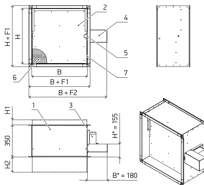
Схема 142. Клапан EI60 (EI90)
