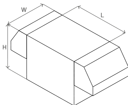
Схема 79. Габаритные размеры внешнего модуля установок WHEEL POLARIS TOP
