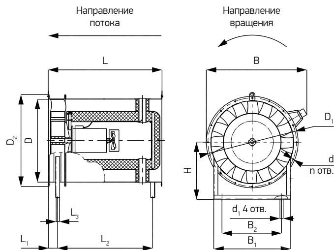
Схема 111. Исполнение SE.400_ F
