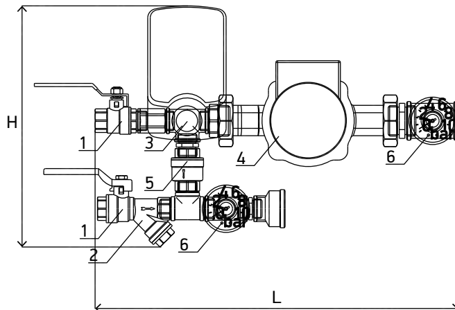
Схема 159. Смесительный узел /MUB...TM
