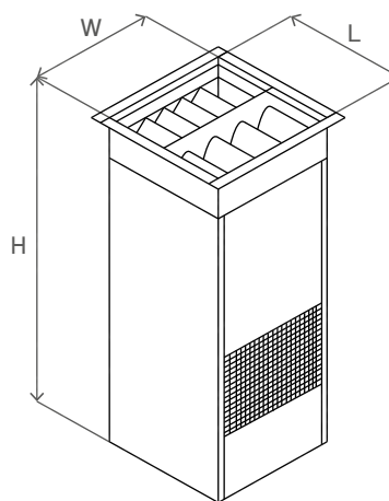
Схема 78. Габаритные размеры внутреннего модуля установок WHEEL SIRIUS TOP
