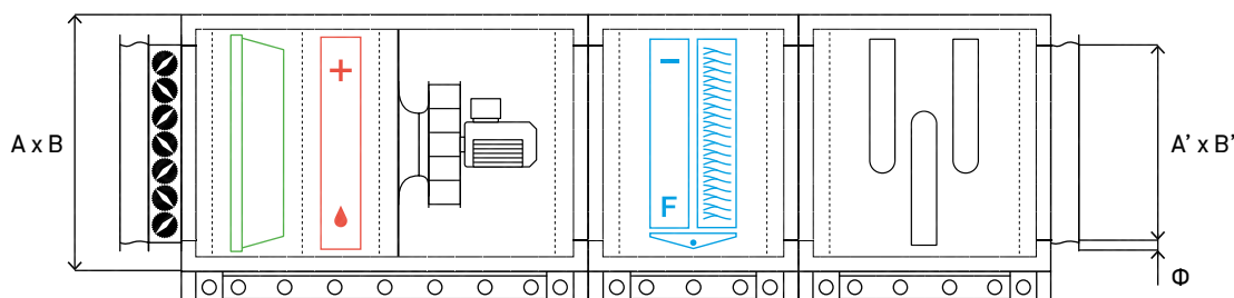
Схема 65. Габаритные размеры установок WHEEL SIRIUS
