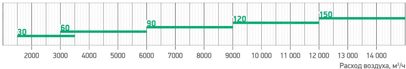
Гр. 72. Рекомендуемые типоразмеры установок WHEEL POLARIS TOP в зависимости от расхода воздуха
