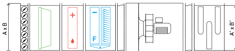
Табл. 230. Габаритно-весовые характеристики элементов установок WHEEL WEGA XP EXPRO
