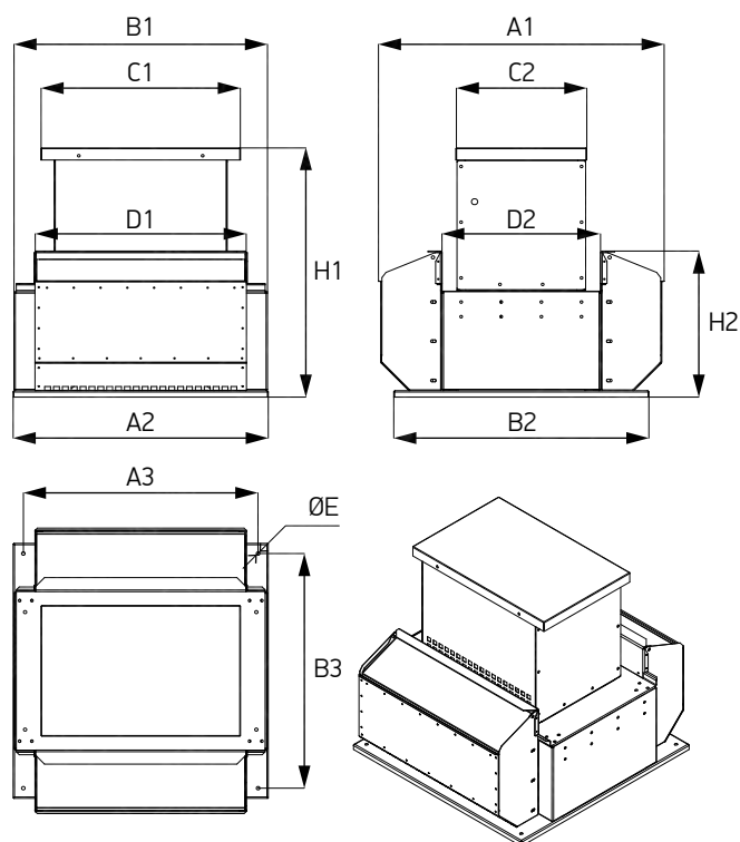
Схема 82. Исполнение с выхлопом вверх WHEEL SHAULA ROOF SE /FPV
