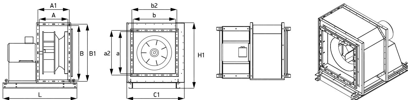
Схема 89. Габаритные и присоединительные характеристики вентиляторов ДУ, ДУВ WHEEL SHAULA FAN SE /FPR (выхлоп вправо, 270°)
