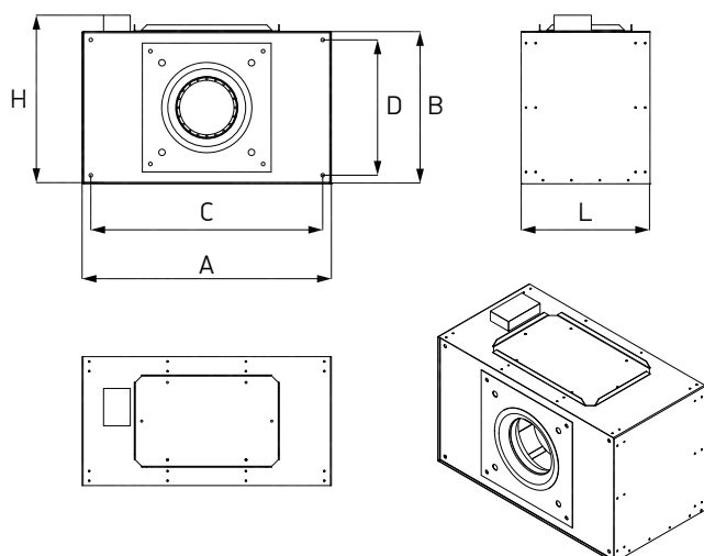
Рис. 3. Габаритные и присоединительные размеры вентиляторов /FEC
