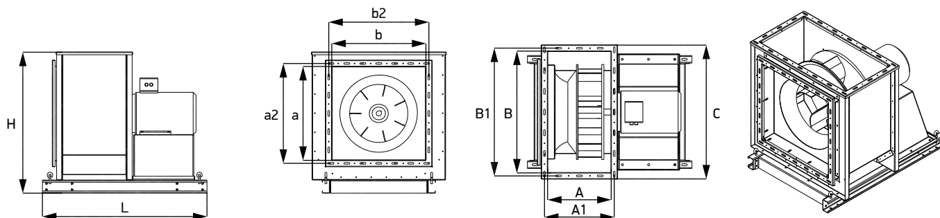
Схема 88. Габаритные и присоединительные характеристики вентиляторов ДУ, ДУВ WHEEL SHAULA FAN SE /FPL (выхлоп влево, 90°)
