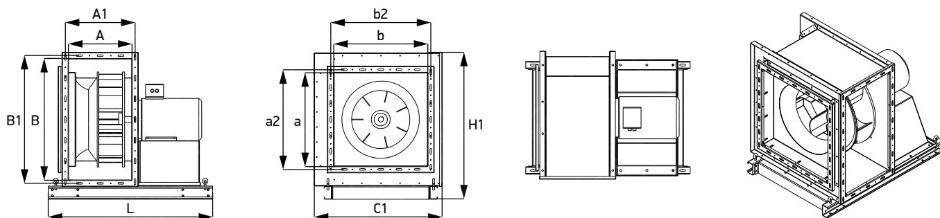
Табл. 111. Габаритные и присоединительные характеристики вентиляторов ДУ WHEEL SHAULA FAN SE /FP_
