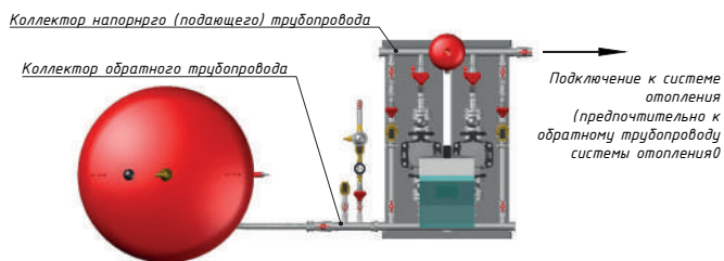
Рис.13 Схема присоединения установки к системе отопления
