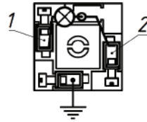
Рис.19 Схема присоединения клапана дренажа
