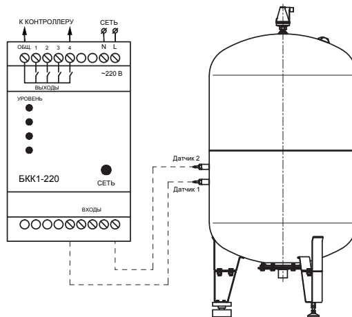
Рис.20 Схема подключения датчика контроля мембраны
