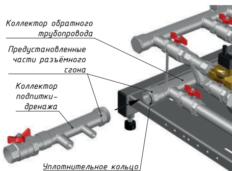
Рис.6 Схема присоединение коллектора подпитки и дренажа
