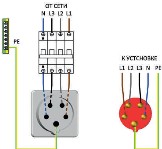
Рис.14 Схема электрическая присоединения установки к сети питания.
