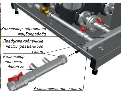
Рис.6 Схема присоединение коллектора подпитки и дренажа
