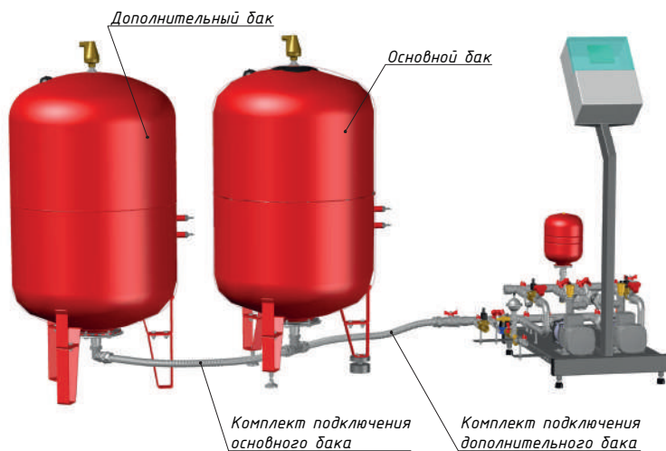
Рис.12 Схема соединения основного и дополнительного бака.
