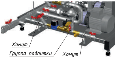
Рис.15 Схема расположения органов управления
