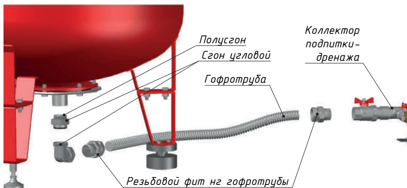
Рис.10 Схема подключения мембранного бака к АУПД
