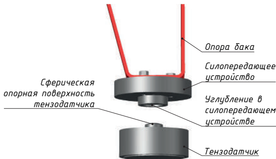
Рис.8 Установка тензодатчика основного мембранного бака.
