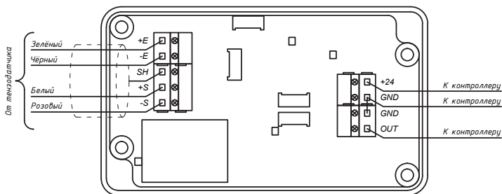
Рис.11 Схема подключения кабеля шкафа управления к нормирующему усилителю НСУ 420-1
