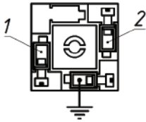
Рис.18 Схема присоединения клапана подпитки
