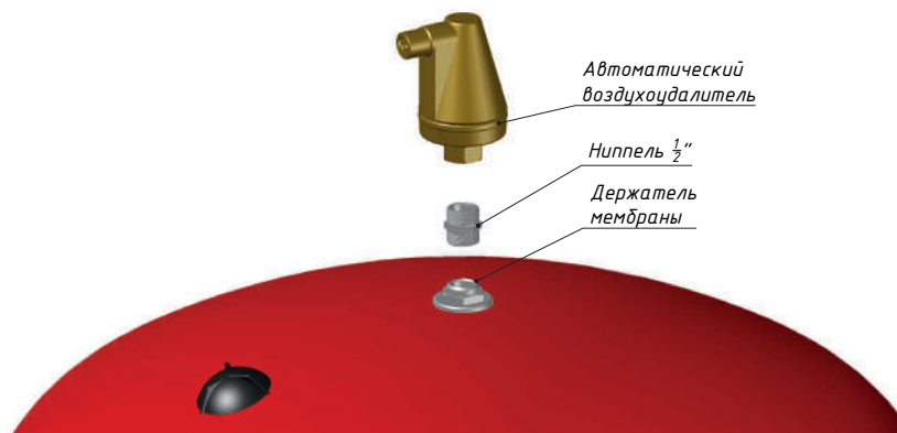
Рис. 7 Схема установки автовоздушника
