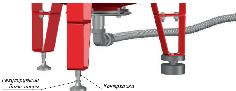
Рис.9 Схема регулирования уровня установки мембранного бака
