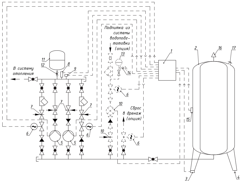
Рис.2 Принципиальная схема установки Westermat
