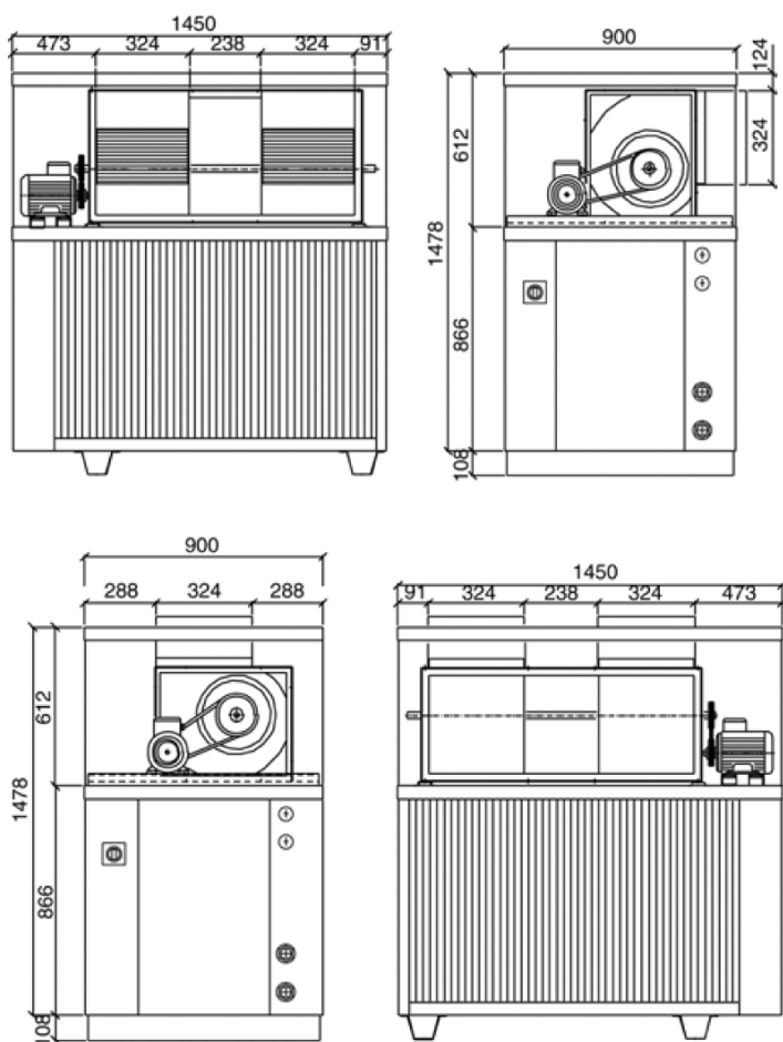
ВЕНТИЛЯТОР С ПРАВОСТОРОННИМ НАГНЕТАНИЕМ ВОЗДУХА
