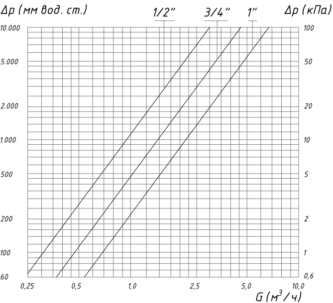
График Kvs клапана Weser PV Compact
