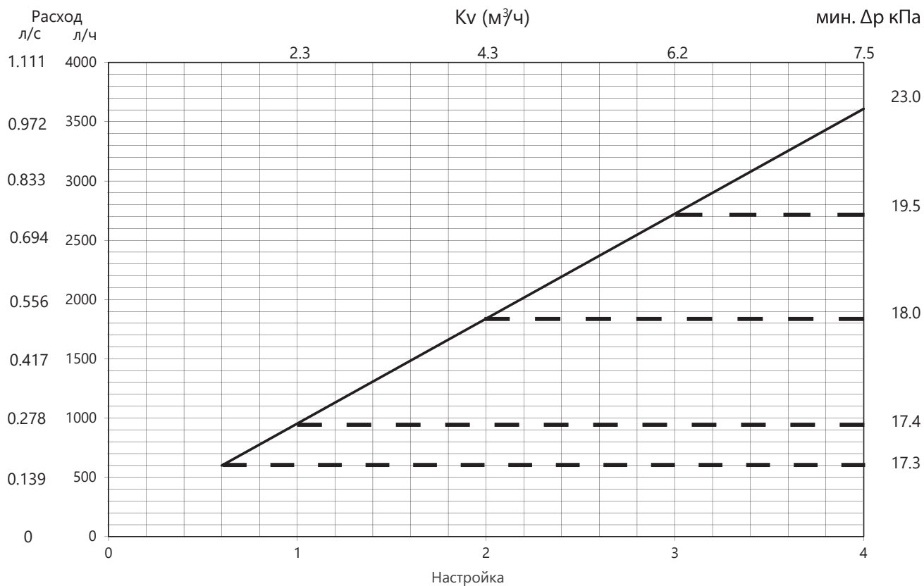
График расхода Frese Optima Compact High 5.5 DN25L
