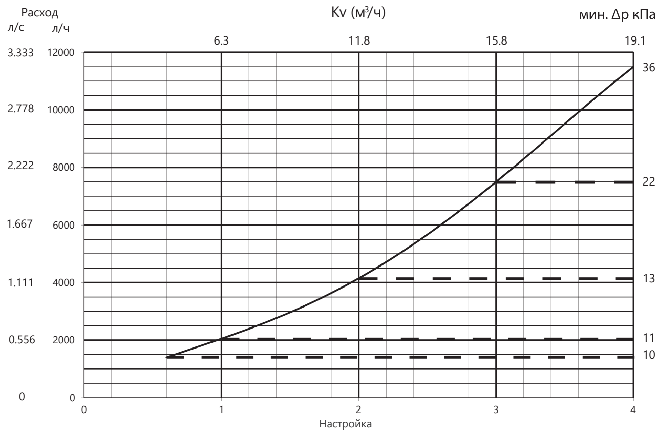
График расхода Frese Optima Compact DN50
