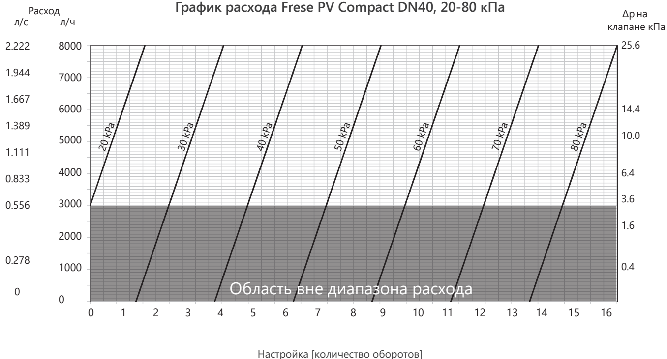
График расхода Frese PV Compact DN40, 20-80 кПа
