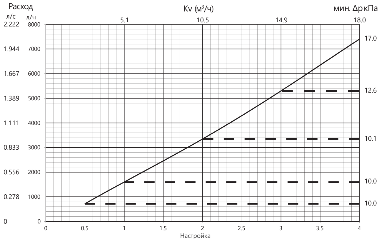
График расхода Frese Sigma Compact DN40
