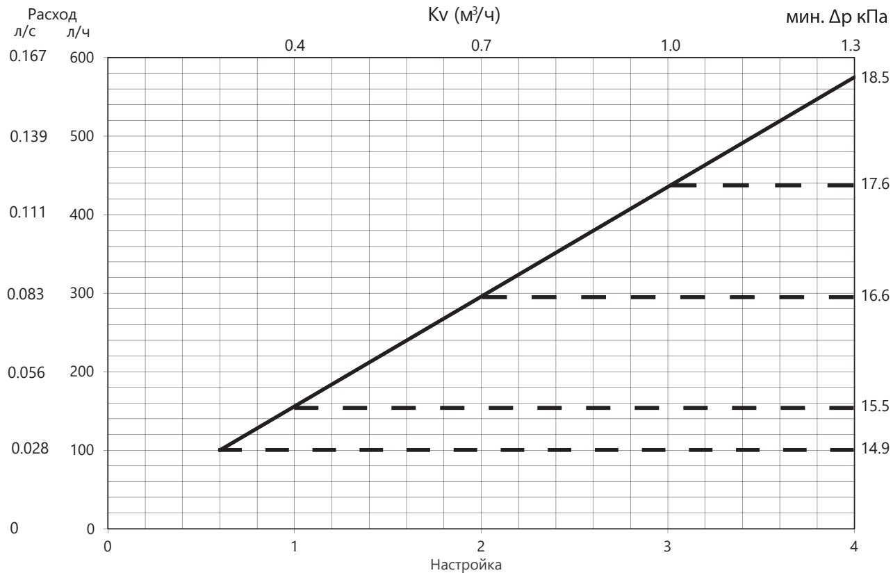
График расхода Frese Optima Compact High 2.5 DN15/20
