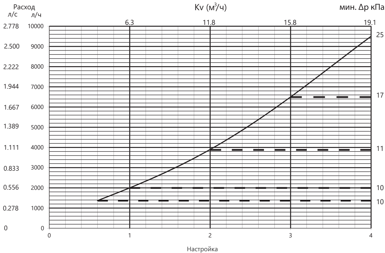
График расхода Frese Optima Compact DN40
