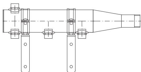
Коллектор сварного типа с конусным переходом
