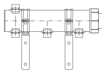
Коллектор резьбового типа
