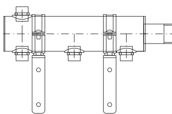
Коллектор сварного типа в компактном исполнении
