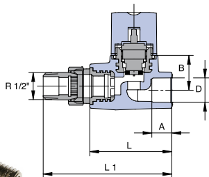
Вентиль радиаторный термостатический прямой
