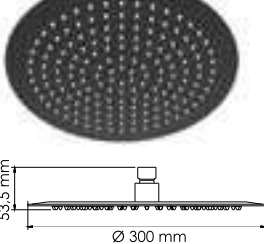
A160 Душевая насадка Нержавеющая сталь, 168 форсунок. Покрытие черный Soft-touch.
