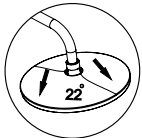
Душевая насадка Душевая насадка для комплекта производится из ABS-пластика. Форсунки из силикона с системой защиты от известковых отложений. Насадка крепится к штанге при помощи шарнирного соединителя, внутрь которого встроен сетчатый аэратор для равномерного распределения воды. Также шарнирный соединитель позволяет менять угол наклона душевой насадки от 0 до 22 градусов.
