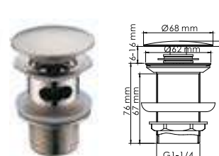
A073 Донный клапан Push-up для раковин с переливом Покрытие «никель».
