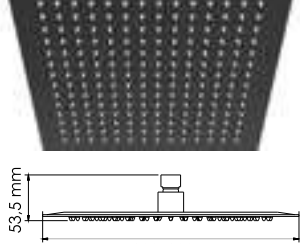
A162 Душевая насадка Нержавеющая сталь, 196 форсунок. Покрытие черный Soft-touch.
