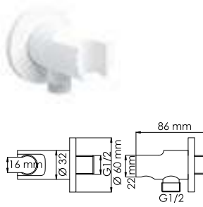
A148 Подключение шланга с настенным держателем лейки. Покрытие белый Soft-touch.
