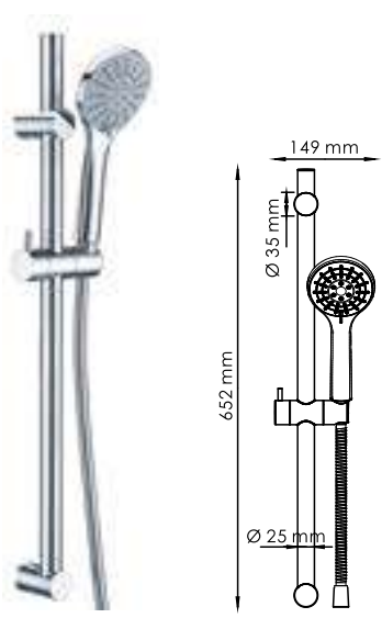
A064 Душевой комплект В комплект входит: - Стойка для душа 652 мм; - Регулируемый держатель лейки; - Шланг металлический 1500 мм; - Лейка 3-функциональная с системой защиты от известковых отложений; - Набор для крепежа.
