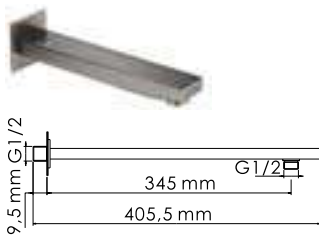
A110 Настенный излив для ванны Покрытие «светая бронза».
