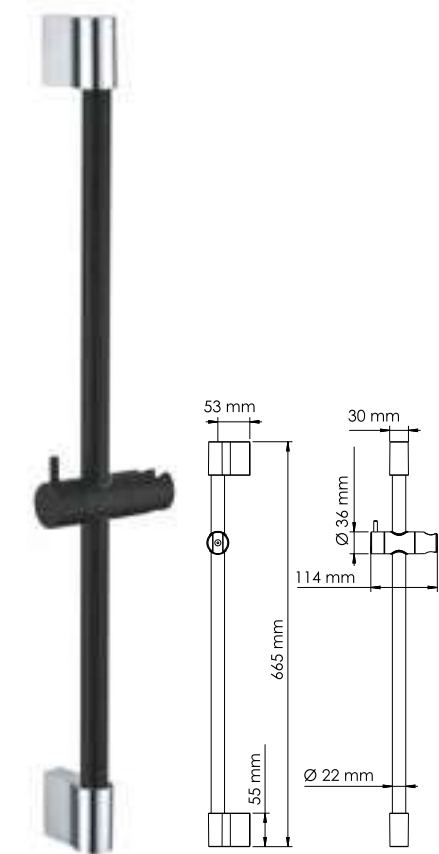
A076 Стойка для душа 66,5 см, Покрытие черный Soft-touch В комплект входит: - Стойка для душа Ø 22 мм; - Регулируемый держатель лейки; - Набор для крепежа.
