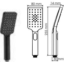
A130 Лейка для душа 3-функциональная с системой защиты от известковых отложений. Покрытие черный Soft-touch.
