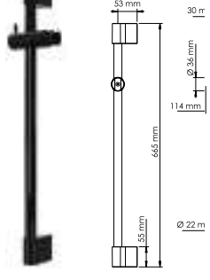
A191 Стойка для душа Нержавеющая сталь, 589 мм Покрытие черный Soft-touch.
