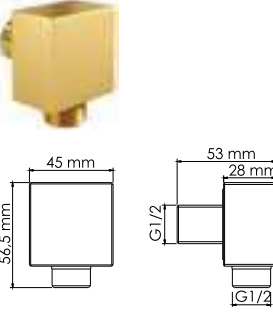
A177 Подключение шланга с настенным держателем лейки. PVD-покрытие «матовое золото».
