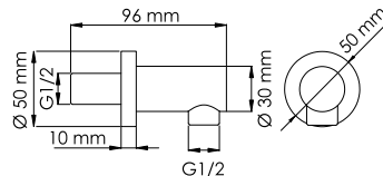
A147 Подключение шланга покрытие белый Soft-touch.
