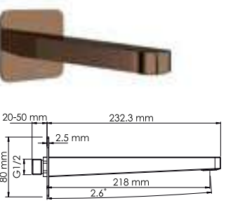
A289 Настенный верхний излив для душа PVD-покрытие «розовое золото».
