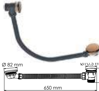
A333 NEW Слив-перелив для ванны, В комплект входит: - Декоративная панель перелива; - Гибкий ПВХ шланг; - Донный клапан. PVD-покрытие «розовое золото».
