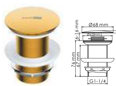
A247 Донный клапан Push-up для раковины без перелива. PVD-покрытие «матовое золото».
