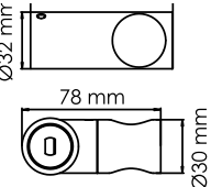
A320 Держатель лейки Поворотный. Покрытие черный Soft-touch.
