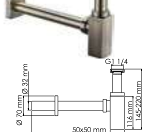
A096 Сифон для раковины Покрытие «светая бронза».
