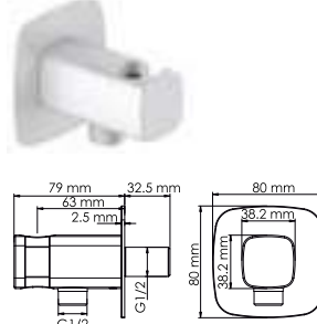
A328 Подключение шланга с настенным держателем лейки. Покрытие белый Soft-touch.
