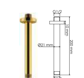
A234 Потолочный излив для душа PVD-покрытие «глянцевое золото».
