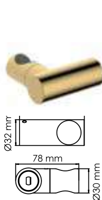
A322 Держатель лейки Поворотный. PVD-покрытие «глянцевое золото».
