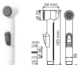
A155 Гигиеническая лейка с фиксатором с системой защиты от известковых отложений. Покрытие белый Soft-touch.
