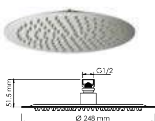
A121 Душевая насадка нержавеющая сталь, 126 форсунок. Покрытие «светая бронза».
