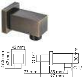
A108 Подключение шланга с настенным держателем лейки. Покрытие «светая бронза».
