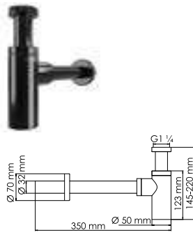
A171 Сифон для раковины PVD-покрытие черный глянец.
