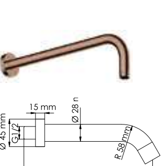
A338 NEW Настенный верхний излив для душа PVD-покрытие «розовое золото».
