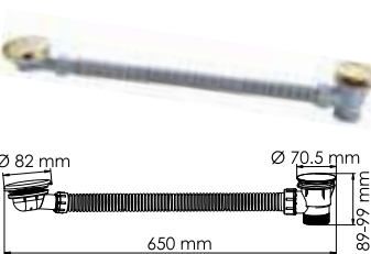
A054 Слив-перелив для ванны. В комплект входит: - Декоративная панель перелива; - Гибкий ПВХ шланг; - Донный клапан. Покрытие «светая бронза».
