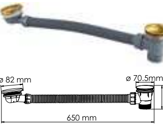
A203 Слив-перелив для ванны, В комплект входит: - Декоративная панель перелива; - Гибкий ПВХ шланг; - Донный клапан. PVD-покрытие «матовое золото».
