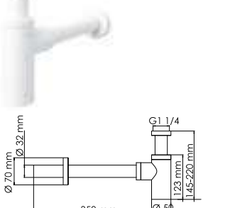
A150 Сифон для раковины Покрытие белый Soft-touch.
