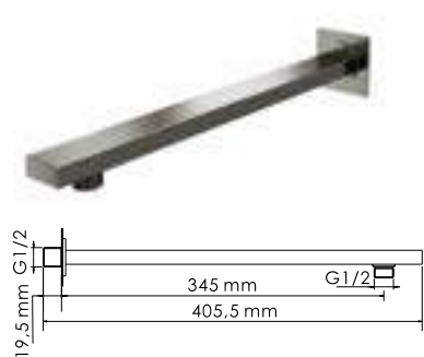
A182 Настенный верхний излив для душа PVD-покрытие «оружейная сталь».
