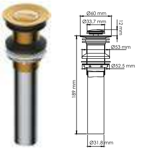
A252 Донный клапан Push-up для раковин без перелива PVD-покрытие «матовое золото».
