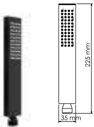
A209 Лейка для душа 1-функциональная с системой защиты от известковых отложений. PVD-покрытие черный глянец.
