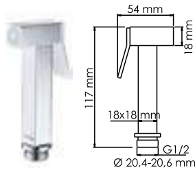
A136 Гигиеническая лейка с фиксатором с системой защиты от известковых отложений.
