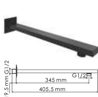
A219 Настенный верхний излив для душа Покрытие черный Soft-touch.
