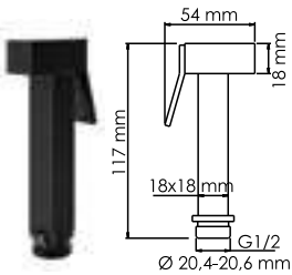
A212 Гигиеническая лейка с фиксатором с системой защиты от известковых отложений. Покрытие черный Soft-touch.
