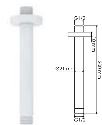
A233 Потолочный излив для душа покрытие белый Soft-touch.
