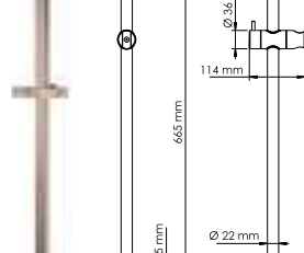
A048 Стойка для душа Нержавеющая сталь, 788 мм Покрытие «светая бронза».
