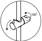
Держатель лейки Держатель с изменяющимся углом поворота лейки 180 градусов. Держатель можно поднять или опустить на любую удобную для Вас высоту, для этого необходимо повернуть рычажок и перемещать по стойке.
