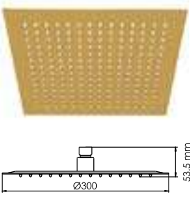
A261 Душевая насадка Нержавеющая сталь, 144 форсунок. PVD-покрытие «глянцевое золото».
