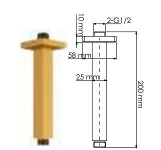
A235 Потолочный излив для душа PVD-покрытие «матовое золото».
