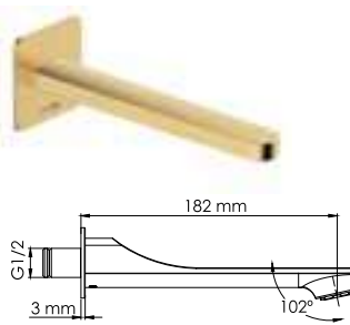
A279 Настенный излив для ванны PVD-покрытие «матовое золото».
