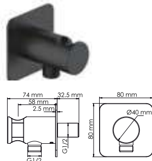
A302 Подключение шланга с настенным держателем Покрытие черный Soft-touch.
