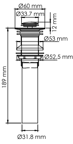
A250 Донный клапан Push-up для раковин без перелива Покрытие черный Soft-touch.
