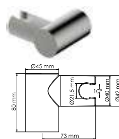
A319 Держатель лейки поворотный. Покрытие «никель».
