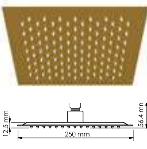
A198 Душевая насадка Нержавеющая сталь, 112 форсунок. PVD-покрытие «матовое золото».
