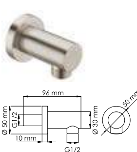
A102 Подключение шланга с настенным держателем лейки. Покрытие «никель».
