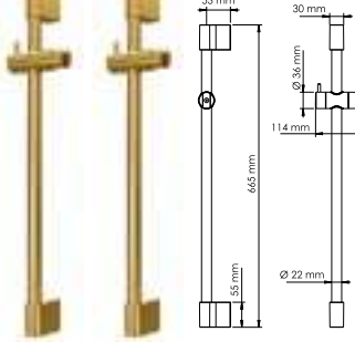
A190, 193 Стойка для душа Нержавеющая сталь, 665 мм PVD-покрытие «глянцевое золото».
