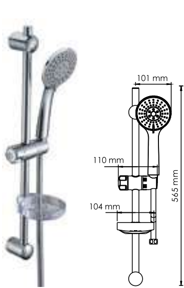
A005 Душевой комплект В комплект входит: - Стойка для душа 565 мм; - Регулируемый держатель лейки; - Мыльница пластиковая, прозрачная; - Шланг металлический 1500 мм; - Лейка 3-функциональная с системой защиты от известковых отложений; - Набор для крепежа.
