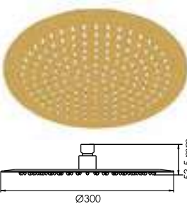
A263 Душевая насадка Нержавеющая сталь, 144 форсунок. PVD-покрытие «глянцевое золото».
