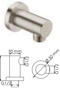
A102 Подключение шланга Покрытие никель
