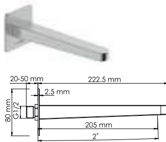
A298 Настенный верхний излив для душа Покрытие «никель».
