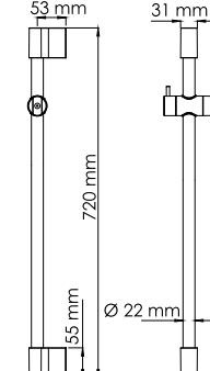
A154 Стойка для душа 72 см, покрытие белый Soft-touch В комплект входит: - Стойка для душа Ø 22 мм; - Регулируемый держатель лейки; - Набор для крепежа.
