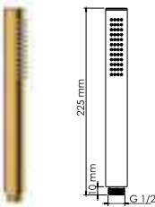
A281 Лейка для душа 1-функциональная с системой защиты от известковых отложений. PVD-покрытие «глянцевое золото».
