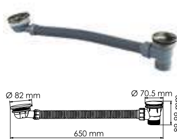
A205 Слив-перелив для ванны Латунь, ПВХ, PVD-покрытие «оружейная сталь».
