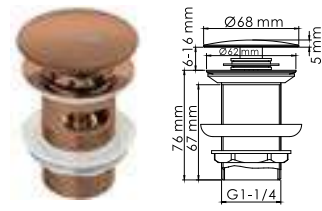
A336 NEW Донный клапан Push-up для раковин с переливом PVD-покрытие «розовое золото».
