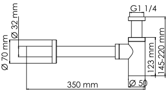
A150 Сифон для раковины покрытие белый Soft-touch.
