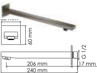
A107 Настенный излив для ванны Покрытие «светая бронза».
