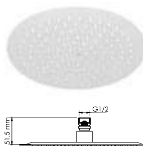
A257 Душевая насадка Нержавеющая сталь, 126 форсунок. Покрытие белый Soft-touch.
