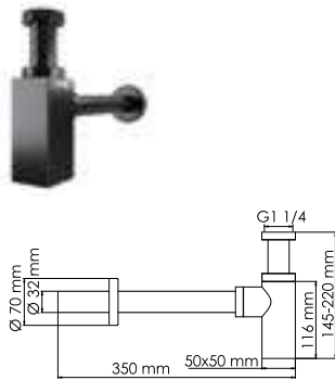
A169 Сифон для раковины Покрытие черный Soft-touch.
