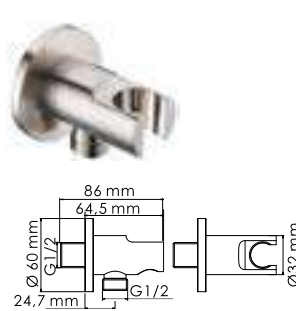
A099 Подключение шланга с настенным держателем лейки. Покрытие «никель».
