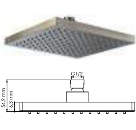
A140 Душевая насадка нержавеющая сталь, 144 форсунок. Покрытие «светая бронза».
