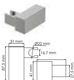
A321 Держатель лейки поворотный. Покрытие «никель».
