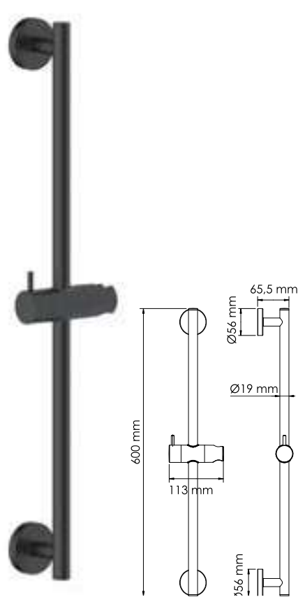
A317 Стойка для душа, 60 см, Покрытие черный Soft-touch В комплект входит: - Стойка для душа Ø 19 мм; - Регулируемый держатель лейки; - Набор для крепежа.
