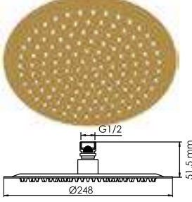
A259 Душевая насадка Нержавеющая сталь, 126 форсунок. PVD-покрытие «матовое золото».
