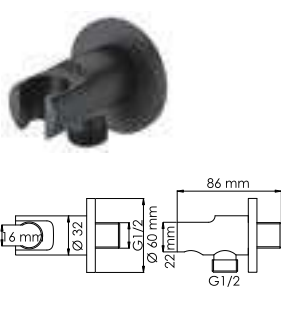
A083 Подключение шланга с настенным держателем Покрытие черный Soft-touch.
