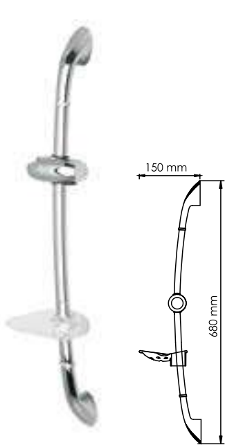
A006 Душевой комплект В комплект входит: - Стойка для душа 680 мм; - Держатель лейки поворотный; - Мыльница пластиковая, прозрачная; - Набор для крепежа.
