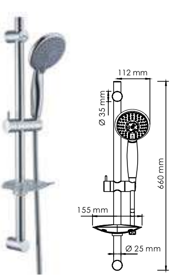
A004 Душевой комплект В комплект входит: - Стойка для душа 660 мм; - Регулируемый держатель лейки; - Мыльница пластиковая, прозрачная; - Шланг металлический 1500 мм; - Лейка 5-функциональная с системой защиты от известковых отложений; - Набор для крепежа.
