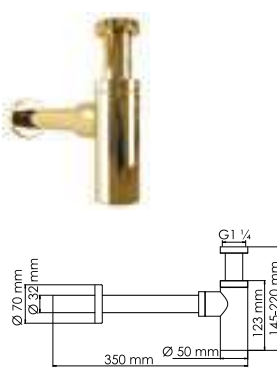
A173 Сифон для раковины PVD-покрытие «глянцевое золото».
