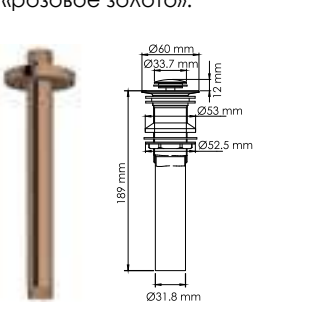
A337 NEW Потолочный излив для душа PVD-покрытие «розовое золото».
