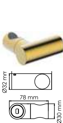
A324 Держатель лейки Поворотный. PVD-покрытие «матовое золото».
