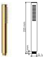
A286 Лейка для душа 1-функциональная с системой защиты от известковых отложений. PVD-покрытие «матовое золото».
