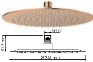
A331 NEW Душевая насадка Нержавеющая сталь, 126 форсунок. PVD-покрытие «розовое золото».
