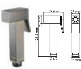
A138 Гигиеническая лейка с фиксатором с системой защиты от известковых отложений. Покрытие «светая бронза».
