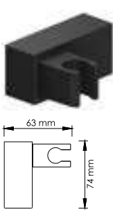
A224 Подключение шланга с настенным держателем PVD-покрытие черный глянец.
