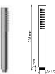
A276 Лейка для душа 1-функциональная с системой защиты от известковых отложений. Покрытие «светая бронза».
