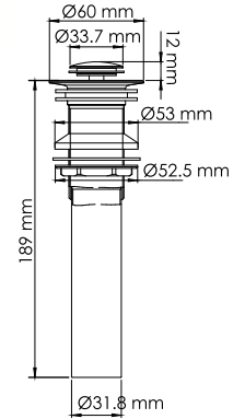
A253 Донный клапан Push-up для раковины без перелива PVD-покрытие «глянцевое золото».
