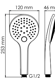
A155 Лейка 3-функциональная с системой защиты от известковых отложений. Покрытие белый Soft-touch.
