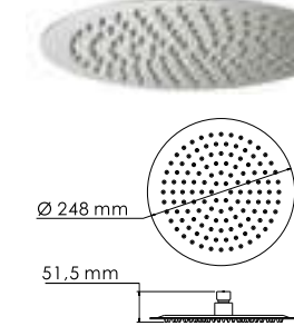
A121 Душевая насадка 126 форсунок Покрытие никель
