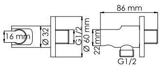
A148 Подключение шланга с настенным держателем лейки. покрытие белый Soft-touch.
