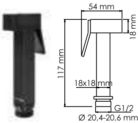
A214 Гигиеническая лейка с фиксатором с системой защиты от известковых отложений. PVD-покрытие черный глянец.
