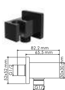
A185 Подключение шланга с настенным держателем PVD-покрытие черный глянец.
