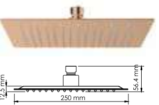
A329 NEW Душевая насадка Нержавеющая сталь, 112 форсунок. PVD-покрытие «розовое золото».
