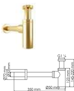
A170 Сифон для раковины PVD-покрытие «матовое золото».
