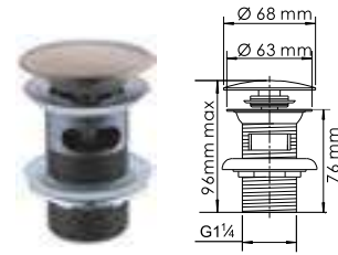
A046 Донный клапан Push-up для раковин с переливом Покрытие «светая бронза».
