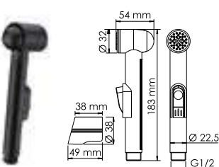
A081 Лейка для душа 1-функциональная с системой защиты от известковых отложений. Покрытие черный Soft-touch.
