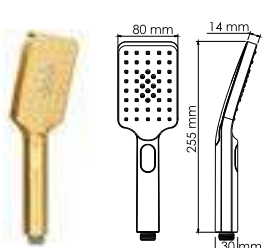
A201 Лейка для душа 3-функциональная с системой защиты от известковых отложений. PVD-покрытие «матовое золото».
