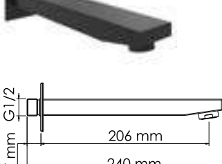
A220 Настенный верхний излив для душа Покрытие черный Soft-touch.
