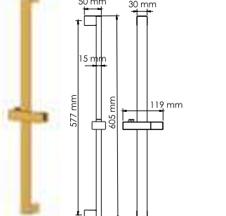
A323 Стойка для душа Нержавеющая сталь, 605 мм PVD-покрыти «матовое золото».
