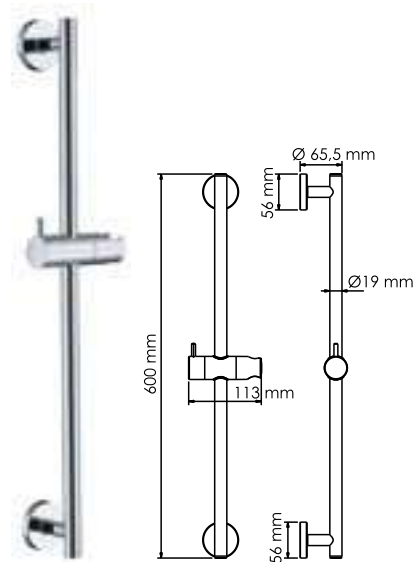
A122 Стойка для душа В комплект входит: - Стойка для душа 600 мм; - Регулируемый держатель лейки; - Набор для крепежа.
