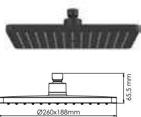
A340 NEW Душевая насадка нержавеющая сталь, 144 форсунок. Покрытие черный Soft-touch.
