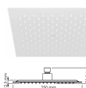
A254 Душевая насадка Нержавеющая сталь, 112 форсунок. Покрытие белый Soft-touch.
