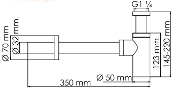
A173 Сифон для раковины PVD-покрытие «глянцевое золото».
