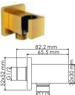
A184 Подключение шланга с настенным держателем лейки. PVD-покрытие «матовое золото».
