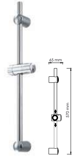
A007 Стойка для душа В комплект входит: - Стойка для душа 570 мм; - Держатель лейки поворотный; - Набор для крепежа.
