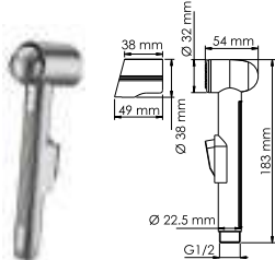
A092 Гигиеническая лейка с фиксатором с системой защиты от известковых отложений. Покрытие «светая бронза».
