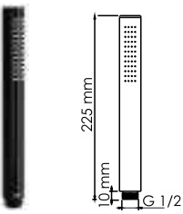
A217 Лейка для душа 1-функциональная с системой защиты от известковых отложений. Покрытие черный Soft-touch.
