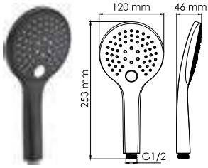
A078 Лейка для душа 3-функциональная с системой защиты от известковых отложений. Покрытие черный Soft-touch.
