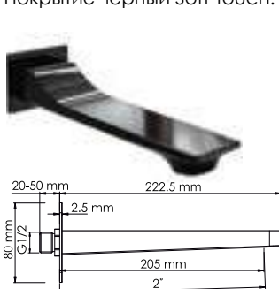
A305 Настенный верхний излив для душа PVD-покрытие черный глянец.
