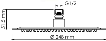
A208 Верхняя душевая насадка Нержавеющая сталь, PVD-покрытие «глянцевое золото». 90 форсунок
