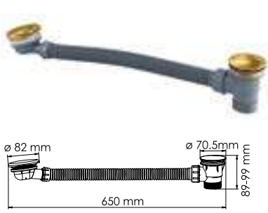
A203 Слив-перелив для ванны Латунь, ПВХ, PVD-покрытие «матовое золото».
