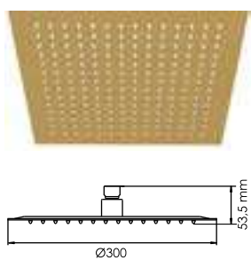
A260 Душевая насадка Нержавеющая сталь, 144 форсунок. PVD-покрытие «матовое золото».
