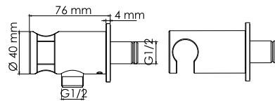
A189 Подключение шланга с настенным держателем лейки. PVD-покрытие «глянцевое золото».
