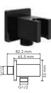
A222 Подключение шланга с настенным держателем PVD-покрытие черный глянец.
