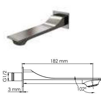
A176 Настенный излив для ванны PVD-покрытие «оружейная сталь».
