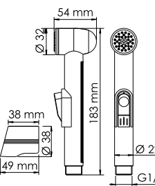
A157 Гигиеническая лейка с фиксатором. покрытие белый Soft-touch.
