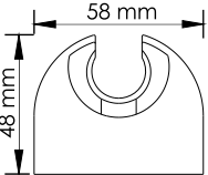
A223 Настенный держатель лейки Фиксированный. Покрытие черный Soft-touch.
