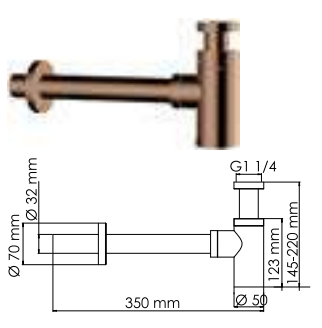
A334 NEW Сифон для раковины PVD-покрытие «розовое золото».
