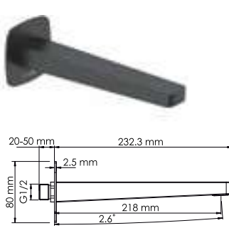
A315 Настенный излив для ванны Покрытие черный Soft-touch.
