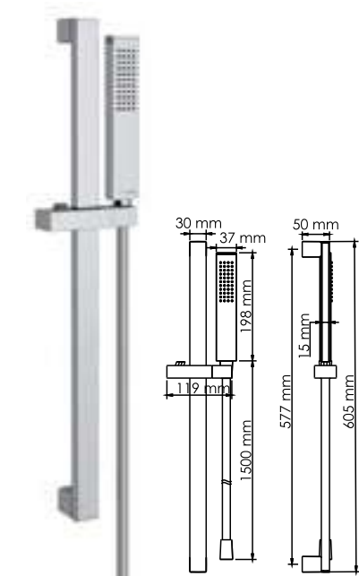
A143 Душевой комплект В комплект входит: - Стойка для душа 605 мм; - Шланг ПВХ 1500 мм; - Лейка 1-функциональная с системой защиты от известковых отложений; - Держатель лейки поворотный; - Набор для крепежа.
