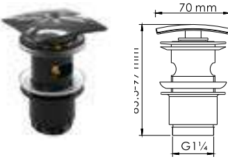
A166 Донный клапан Push-up для раковин без перелива PVD-покрытие черный глянец.
