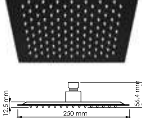
A199 Душевая насадка Нержавеющая сталь, 112 форсунок. PVD-покрытие черный глянец.
