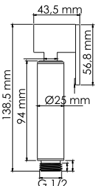
A232 Гигиеническая лейка с фиксатором. покрытие белый Soft-touch.
