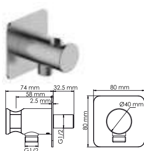
A275 Подключение шланга с настенным держателем лейки. Покрытие «никель».
