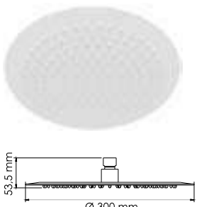
A161 Душевая насадка Нержавеющая сталь, 168 форсунок. Покрытие белый Soft-touch.
