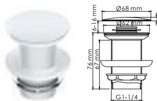
A246 Донный клапан Push-up для раковин с переливом Покрытие белый Soft-touch.
