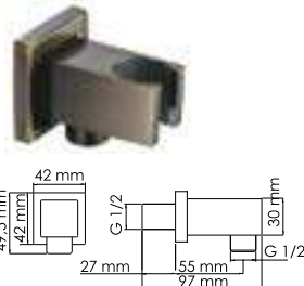
A109 Подключение шланга с настенным держателем лейки. Покрытие «светая бронза».
