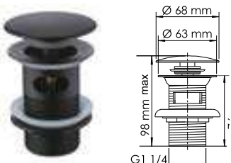
A080 Донный клапан Push-up для раковин с переливом Покрытие черный Soft-touch.
