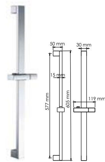
A123 Стойка для душа В комплект входит: - Стойка для душа 605 мм; - Регулируемый держатель лейки; - Набор для крепежа.
