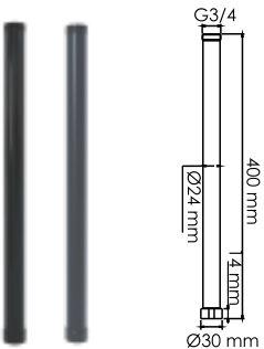
A226, 210 Удлинитель для душевой системы Нержавеющая сталь, PVD-покрытие черный глянец. Покрытие черный Soft-touch.
