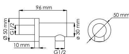
A188 Подключение шланга PVD-покрытие «глянцевое золото».
