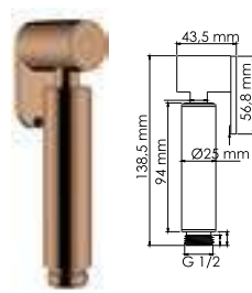
A335 NEW Гигиеническая лейка с фиксатором с системой защиты от известковых отложений. PVD-покрытие «розовое золото».
