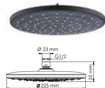
A077 Душевая насадка ABS-пластик, 76 форсунок Покрытие черный Soft-touch.
