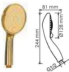
A207 Лейка для душа 1-функциональная с системой защиты от известковых отложений. PVD-покрытие «глянцевое золото».
