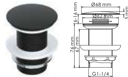
A245 Донный клапан Push-up для раковин без перелива. Покрытие черный Soft-touch.
