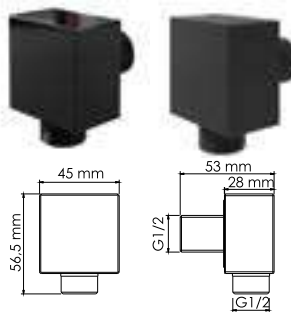
A178, A221 Подключение шланга с настенным держателем PVD-покрытие черный глянец. Покрытие черный Soft-touch.
