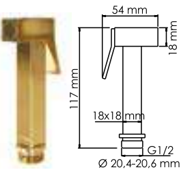
A216 Лейка для душа 1-функциональная с системой защиты от известковых отложений. PVD-покрытие «глянцевое золото».
