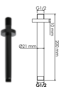
A151 Потолочный излив для душа Покрытие черный Soft-touch.
