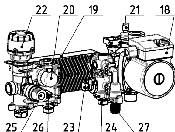
Рис. 10. Общая схема и основные элементы котла
