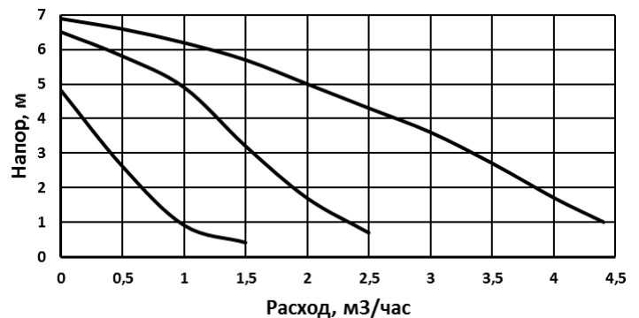
Рис. 13. Напорная харктеристика насоса.
