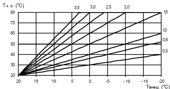
Рис. 3 График зависимости температуры в контуре отопления от внешней температуры при комнатной температуре 20 °С
