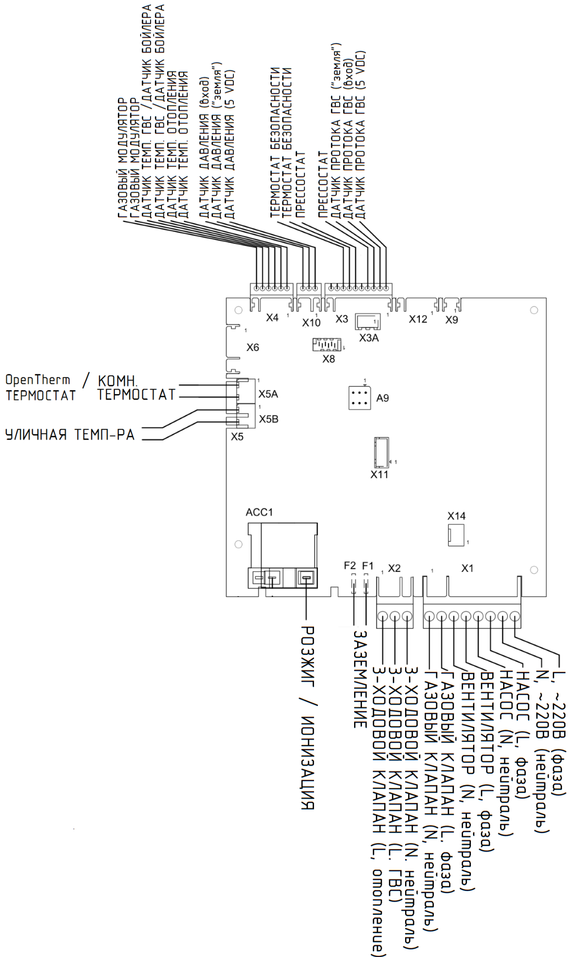
Рис. 14. Электрическая схема
