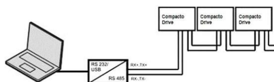
Последовательное подключение
