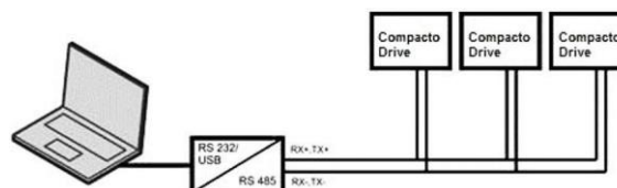
Параллельное подключение
