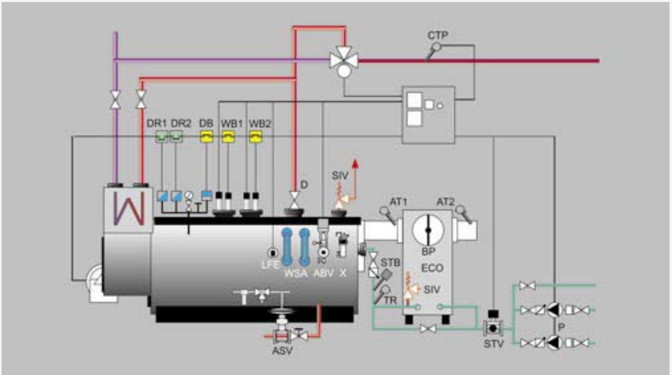
Паровой котел высокого давления серии Vitomax 200 HS, оснащенный пароперегревателем
