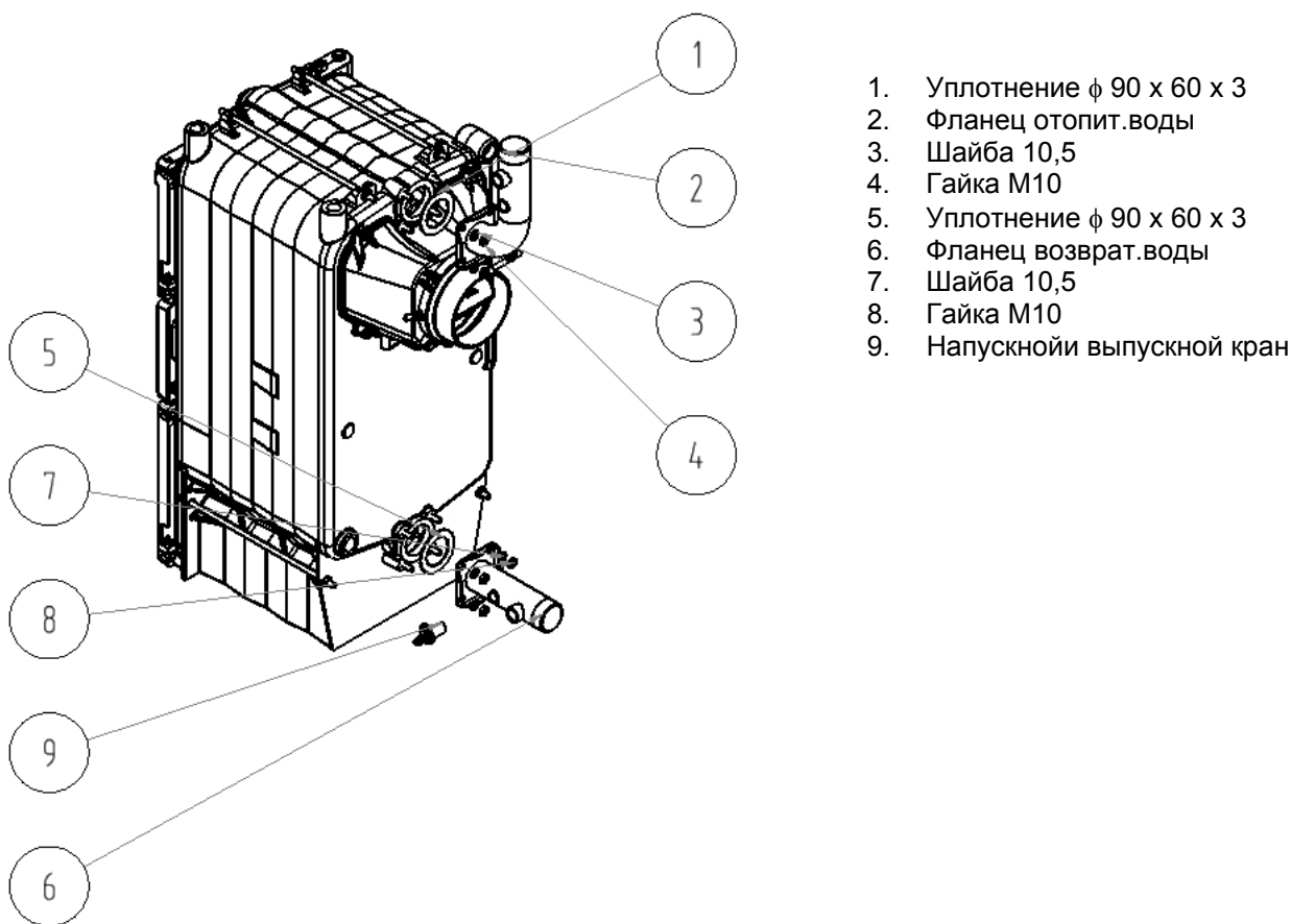
Рис. № 11 Установка котельного корпуса
