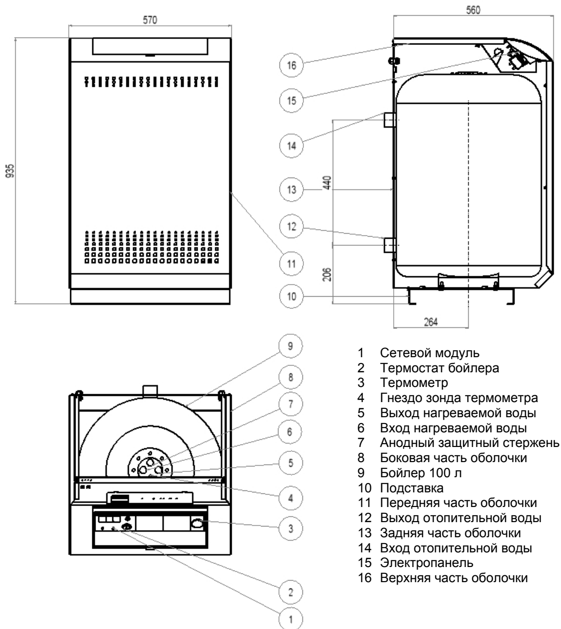
Рис. 1 Состав бойлера VIADRUS OV 100 L (размеры в мм)
