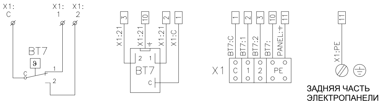
Контурная схема OV 100 L
