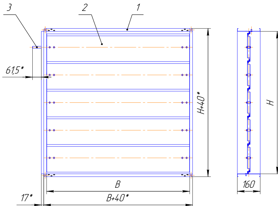
Рисунок А1. Клапан «Канал-РЕГУЛЯР» 1 – корпус, 2 – лопатка, 3 – шток для исполнительного механизма
