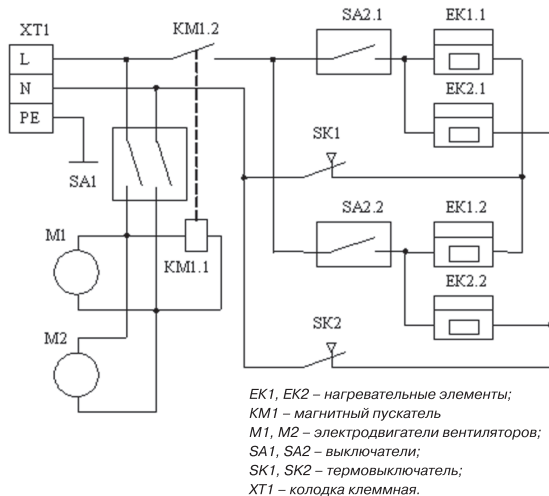
Рис. 3. Схема электрическая НТ 508
