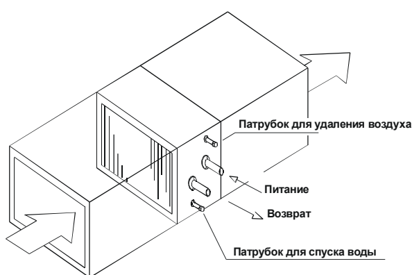
Питание обменника с патрубками нагревателя с правой стороны
