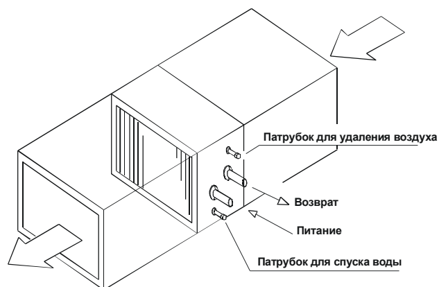
Питание обменника с патрубками нагревателя с левой стороны
