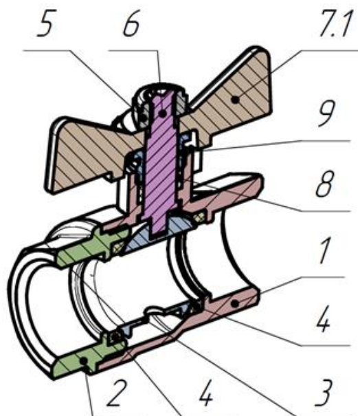
Кран с рукояткой-бабочкой
