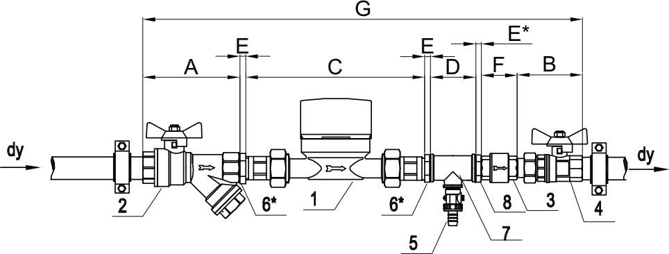
ГАБАРИТНЫЙ ЧЕРТЕЖ
