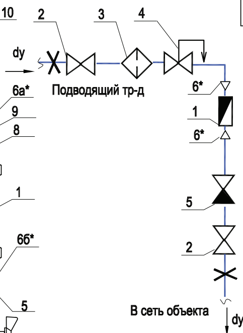
СХЕМА
