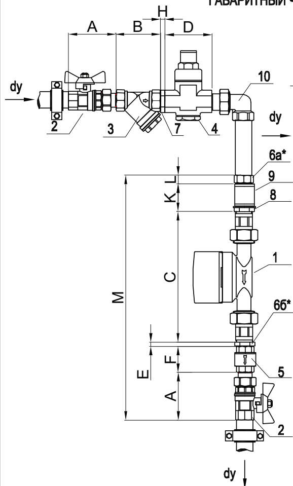
ГАБАРИТНЫЙ ЧЕРТЕЖ
