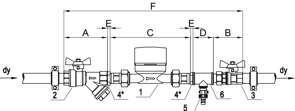
ГАБАРИТНЫЙ ЧЕРТЕЖ
