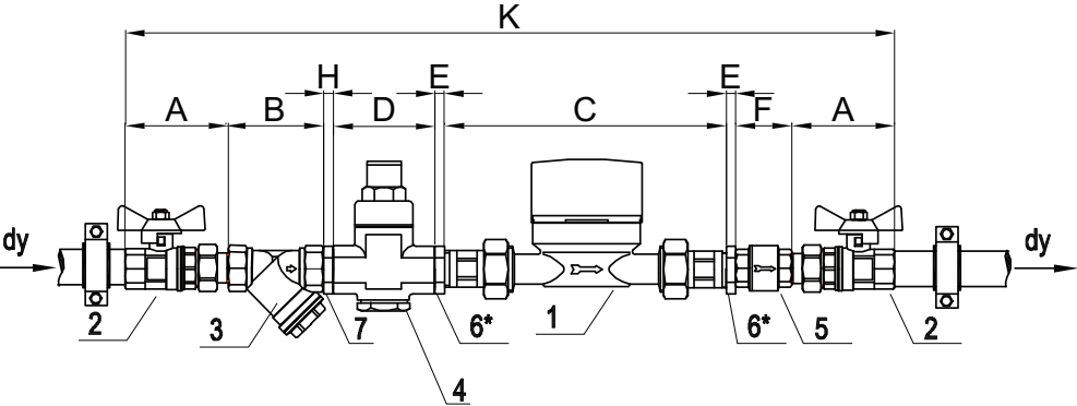
ГАБАРИТНЫЙ ЧЕРТЕЖ
