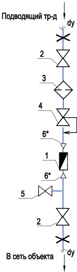
СХЕМА
