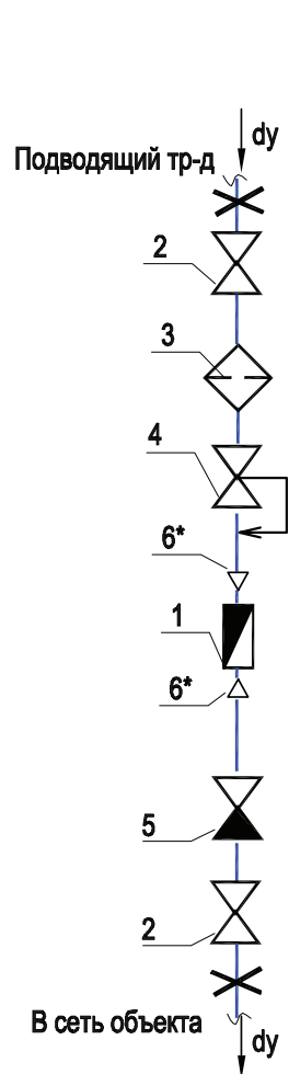
СХЕМА
