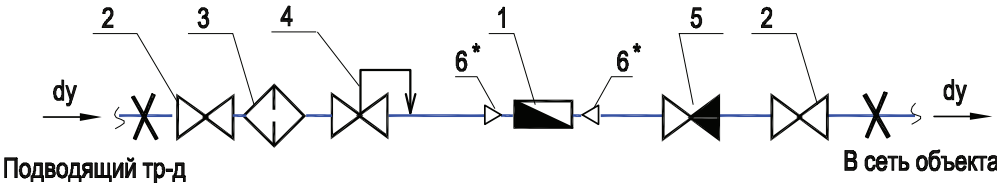
СХЕМА
