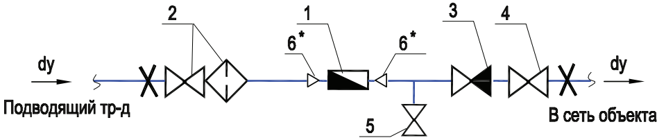
СХЕМА
