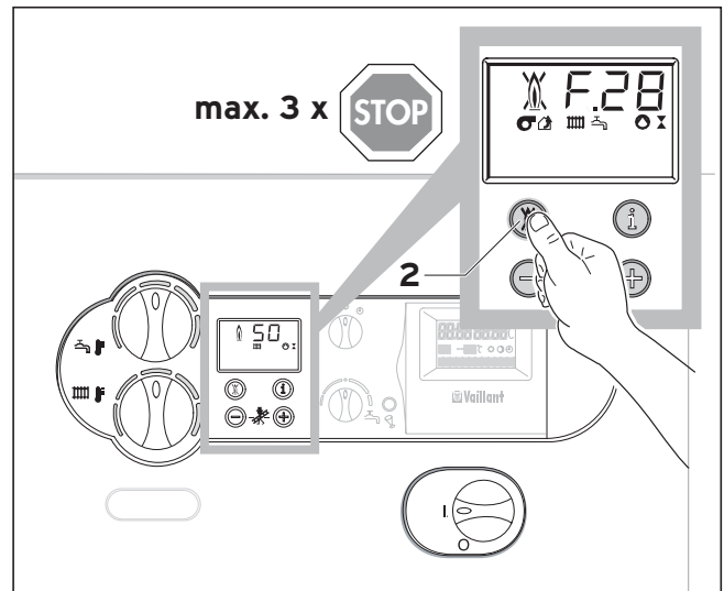
Fig. 5.1 Resetarea avariei
