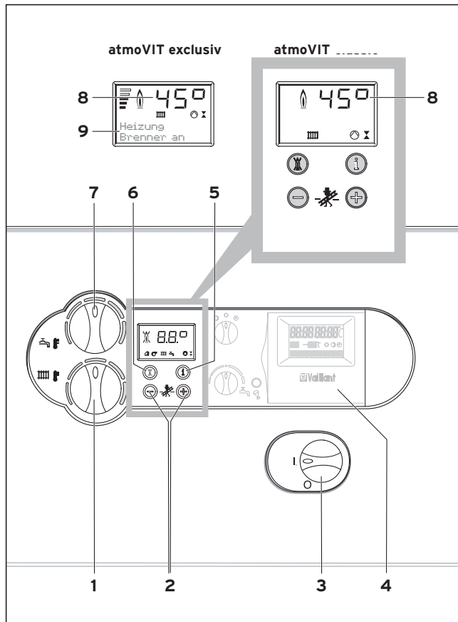
Рис. 4.3 Органы управления
