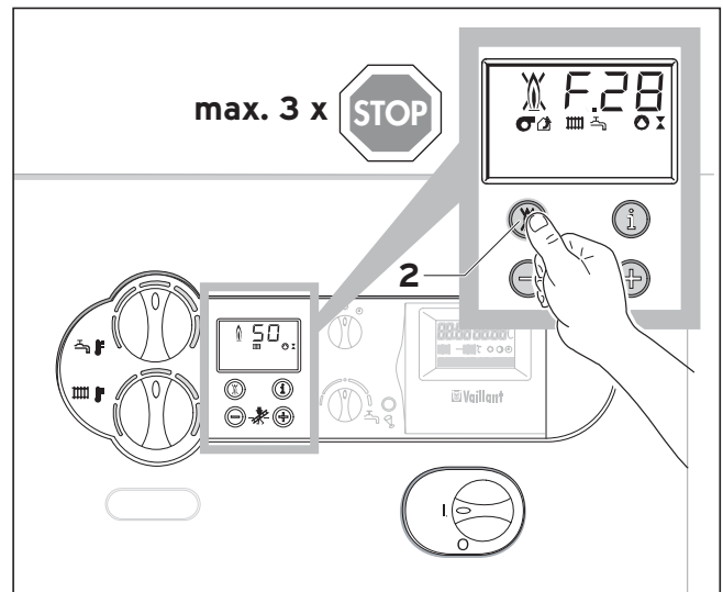
Slika 5.1 Deblokiranje
