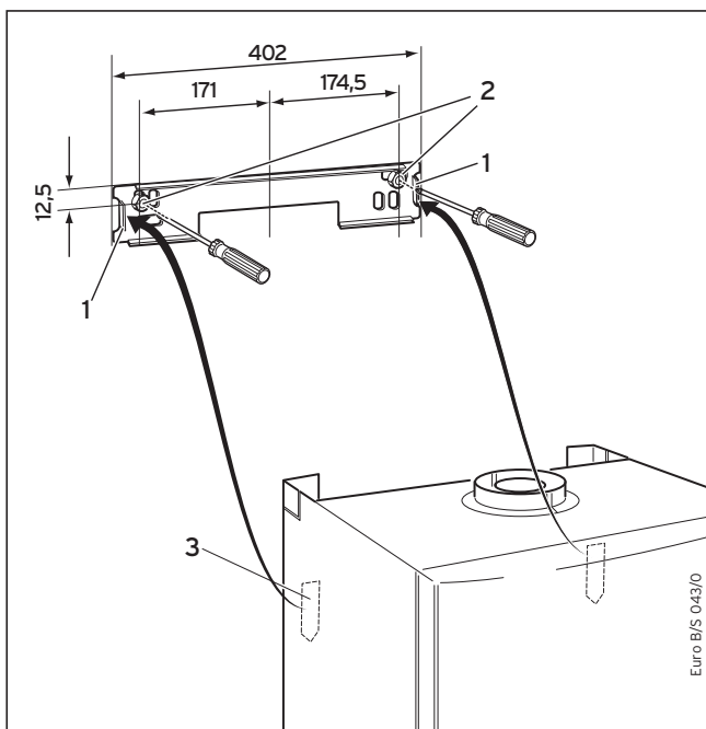
Рис. 3.6 Навеска аппарата
