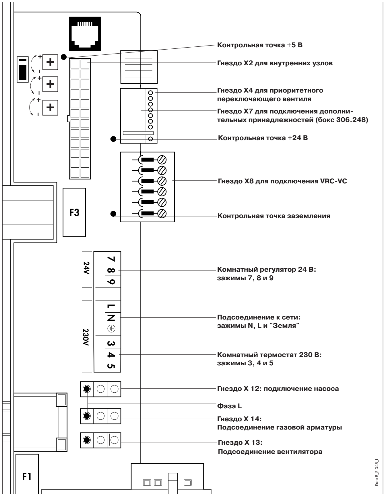
Рис. 3.14 Схема электрических соединений
