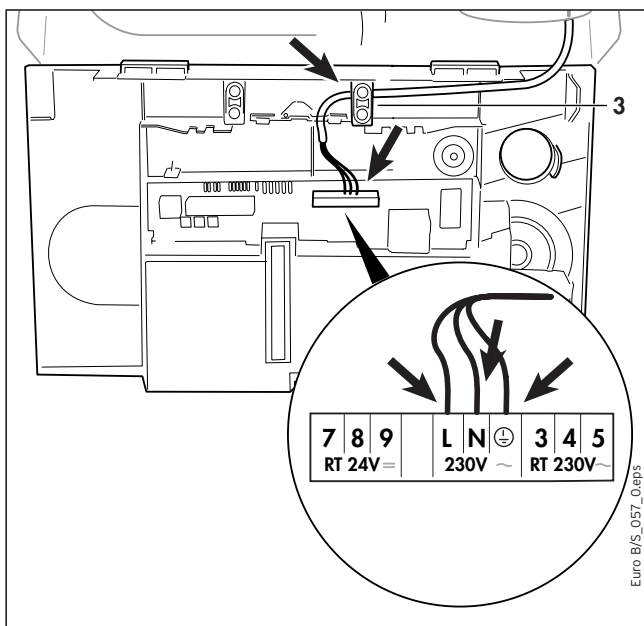
Рис. 3.13 Прокладка кабеля
