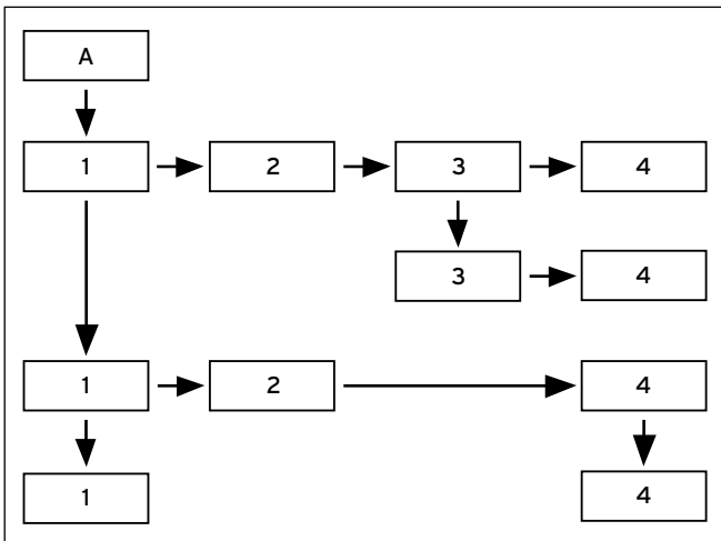
Рис. 3.2 Структура меню
