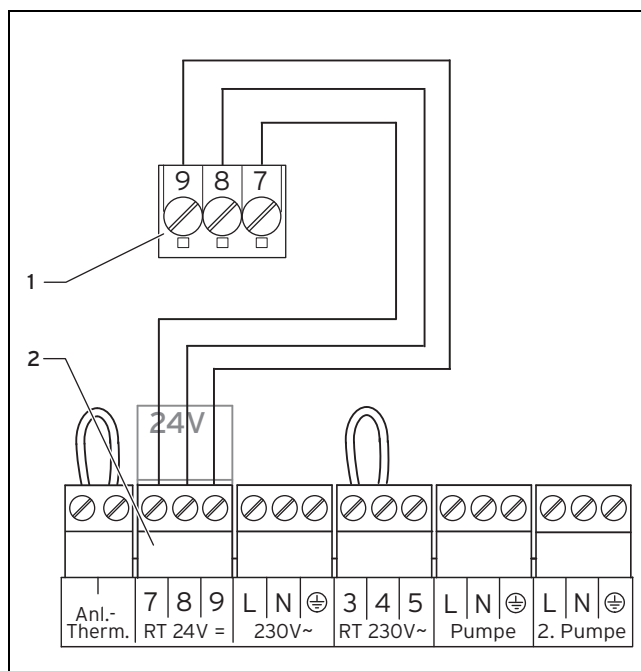
Рисунок 5.1: Подсоединение регулятора
