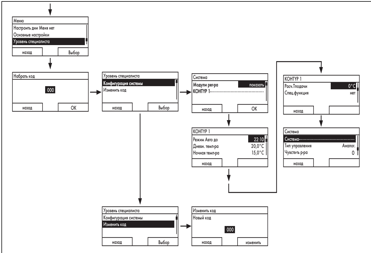
7.1: Структура меню
