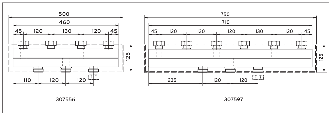
Рис. 1 Размерный чертёж
