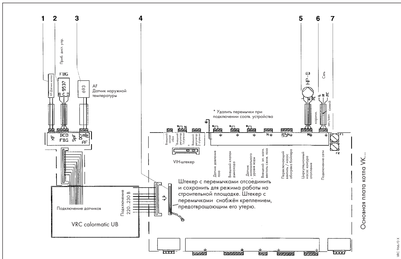
Рис. 4.1 Схема электрических соединений УК...
